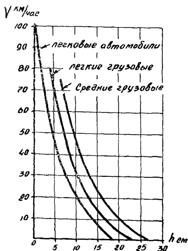
Р и с. 1. Зависимость скорости движения автомобилей от толщины неупругого слоя снега
