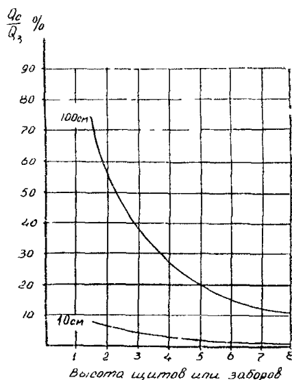
Рис. 38. Однорядные щиты и заборы
