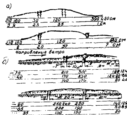
Р и с. 55. Профили снежных отложений у посадок разрывных конструкций
