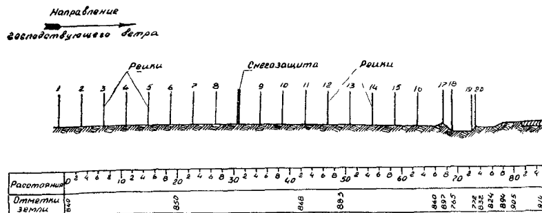
Р и с. 7 3. Пример установки реек на поперечнике снегомерного пункта
