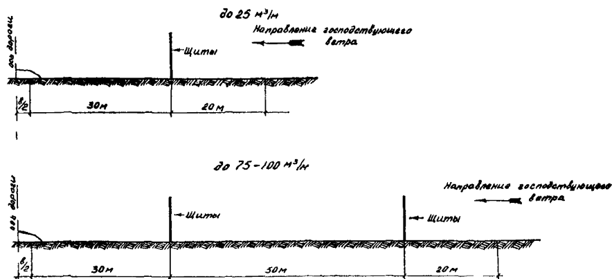
Р и с. 75. Расположение щитовых линий при объемах снегоотложений до 100 м³/м
