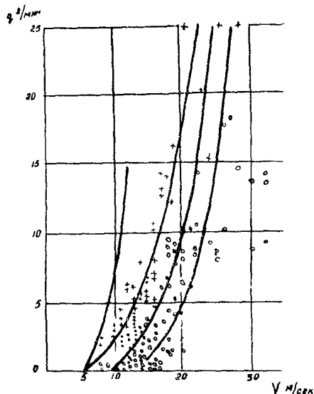
Рис. 5. Зависимость интенсивности низовой метелли от скорости ветра
