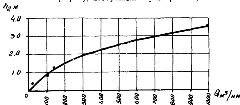
Рис. 34. Превышение бровки незаносимой насыпи над поверхностью образующегося снежного покрова в зависимости от объема снегоприноса
