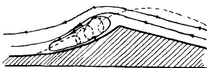
Р и с. 2 4. Образование на подветренном склоне возвышенности зоны циркуляции
