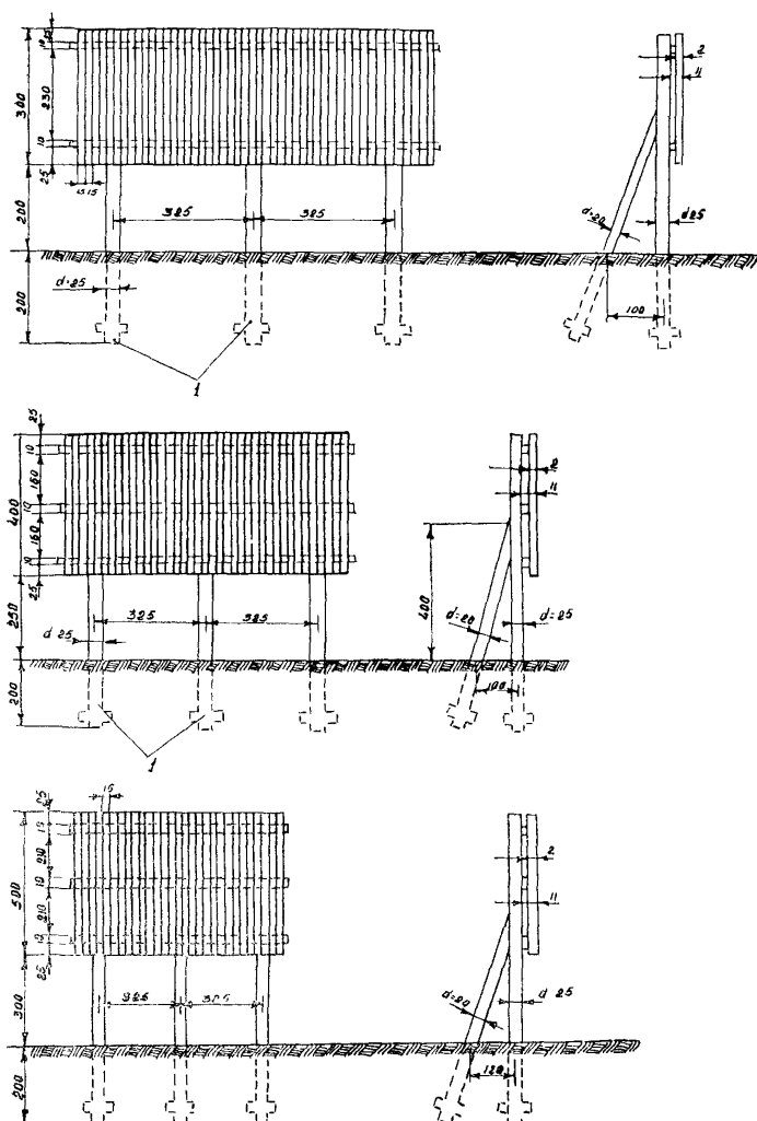
Р и с. 3 5. Рекомендуемые типы снегопередующих заборов (по данным Г. В. Бялобжеского, 1966 г.)
