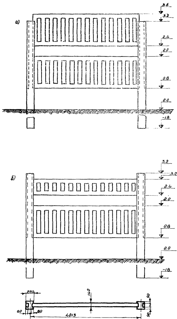
Р и с. 48. Двухпанельный железобетонный забор
