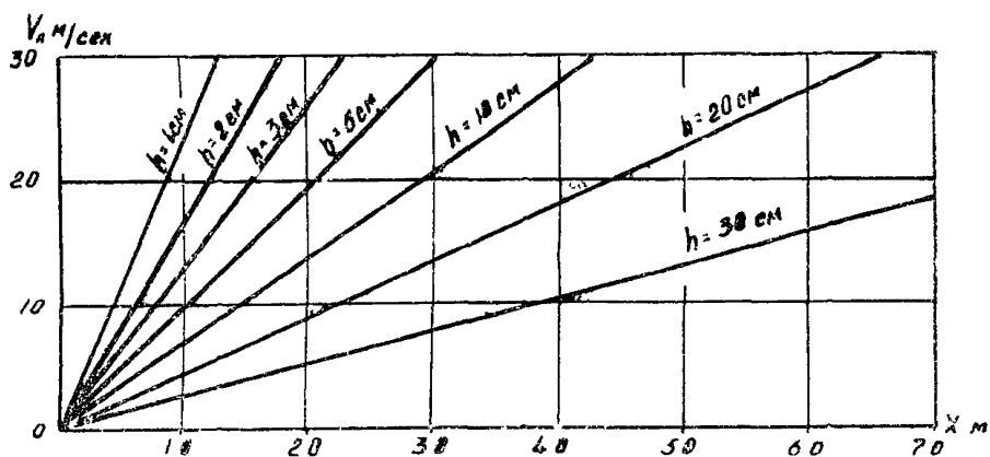
Р и с. 13. Графики расстояний, пролетаемых снежинками при падении в зависимости от начальной скорости V_1 и высоты h
