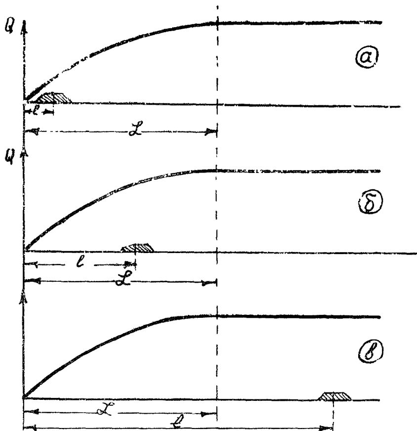
Р и с. 33. Расположение дороги по отношению к границам снегoпереноса
