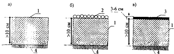
Рис. 2. Схемы конструкций дорожных одежд:
