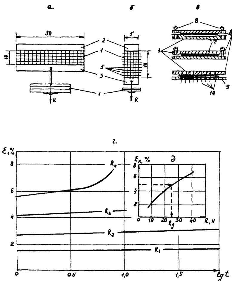
Рис. I. Испытание синтетических материалов на растяжение: а, б, в - схемы нагружения; г, д - результаты испытаний
