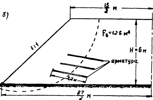
Рис. I. К определению технико-экономической эффективности мероприятий по повышению общей устойчивости откосов
