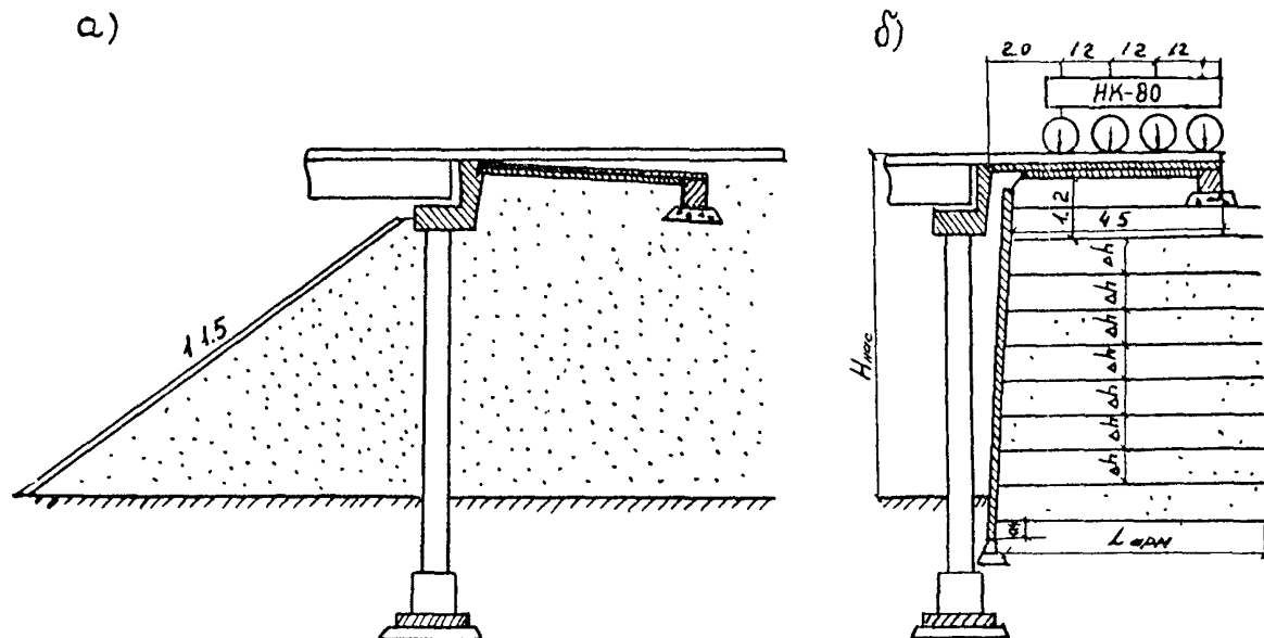
Рис. 3.1. Сравнение типовой конструкции конуса с армогрунтовой конструкцией с подпорной стенкой:
