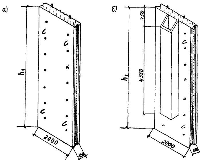
Рис. 3.3. Конструкция блоков подпорной стенки:
