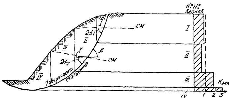
Рис. 2.3. Схема к расчету армированного откоса
