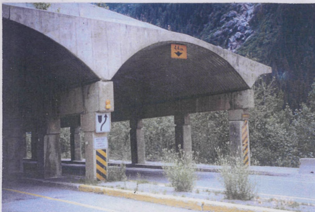
Фото 4. Лавинозащитная галерея со сводом из ГМК
