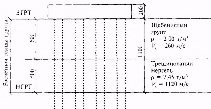
Рис. 5.3. Схема грунтового основания опоры № 9
