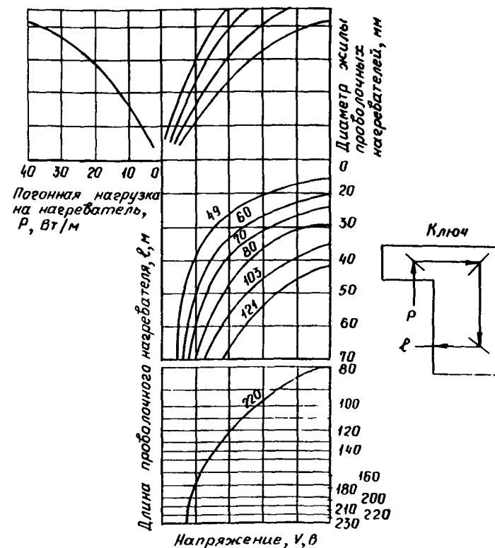
Рис. 3. Номограмма для определения длины проволочных нагревателей
