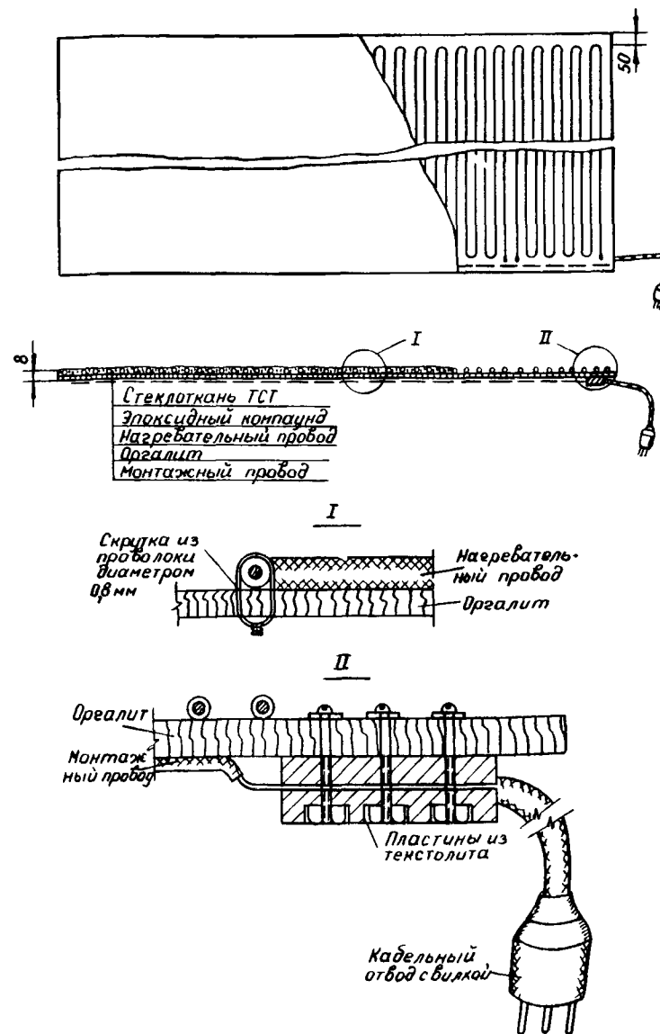
Рис. 1. Гибкий плоский элемент (ГЭП)
