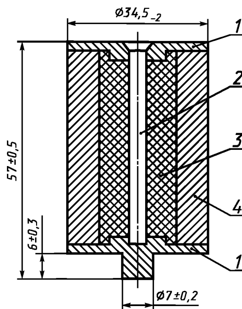
Типоразмер DIV
