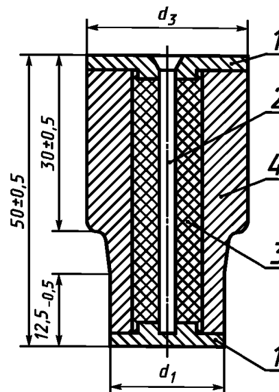
Типоразмеры DII, DIII
