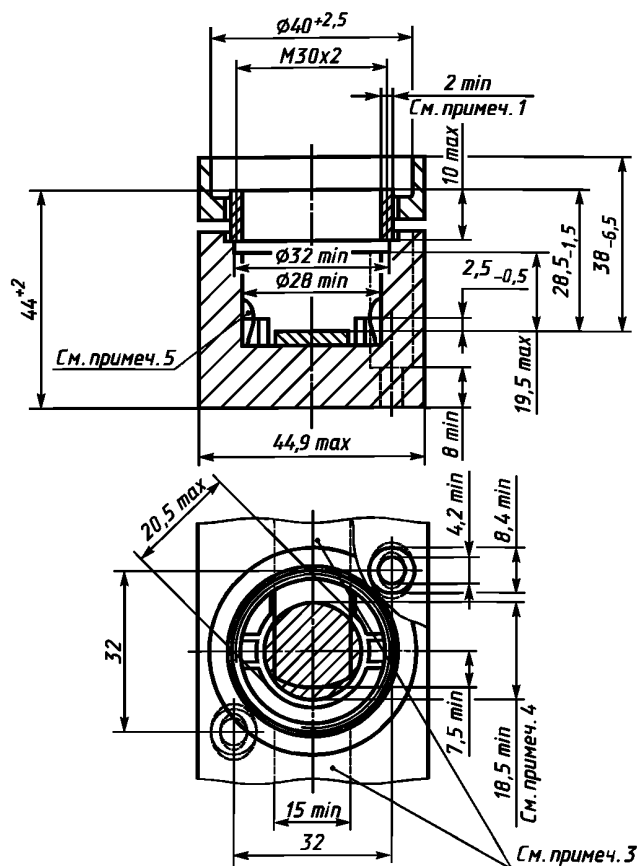
Типоразмер D03
