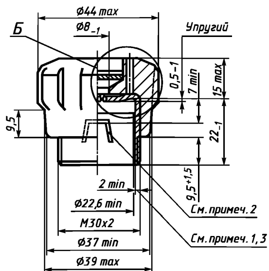
Типоразмер D03
