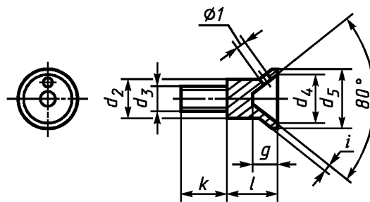
Втулка
