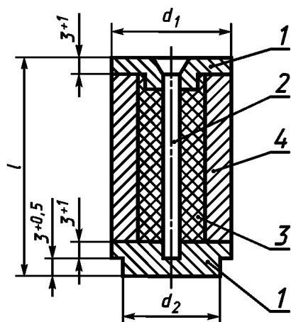
Типоразмеры D01—D03
