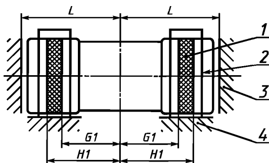
Основание типа А
