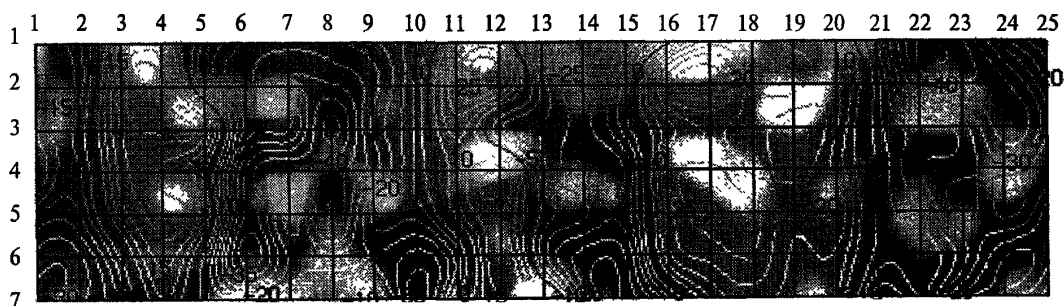
Рисунок К.1 — Пример изображения карты РГМН с областями остаточных пластических деформаций (гофры) конструкции на дисплее ПЭВМ оператора (области между 2—5, 10—13 и 15—21 вертикальными координатными линиями, области остаточных пластических деформаций оконтурены изострессами со значением 0 — на дисплее ПЭВМ красные линии)
