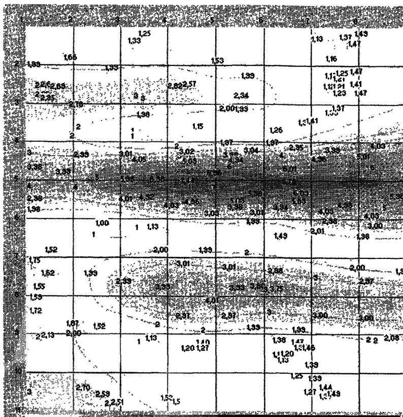
Рисунок И.1 — Пример изображения карты КМН в окрестности сварного шва конструкции на дисплее ПЭВМ оператора
