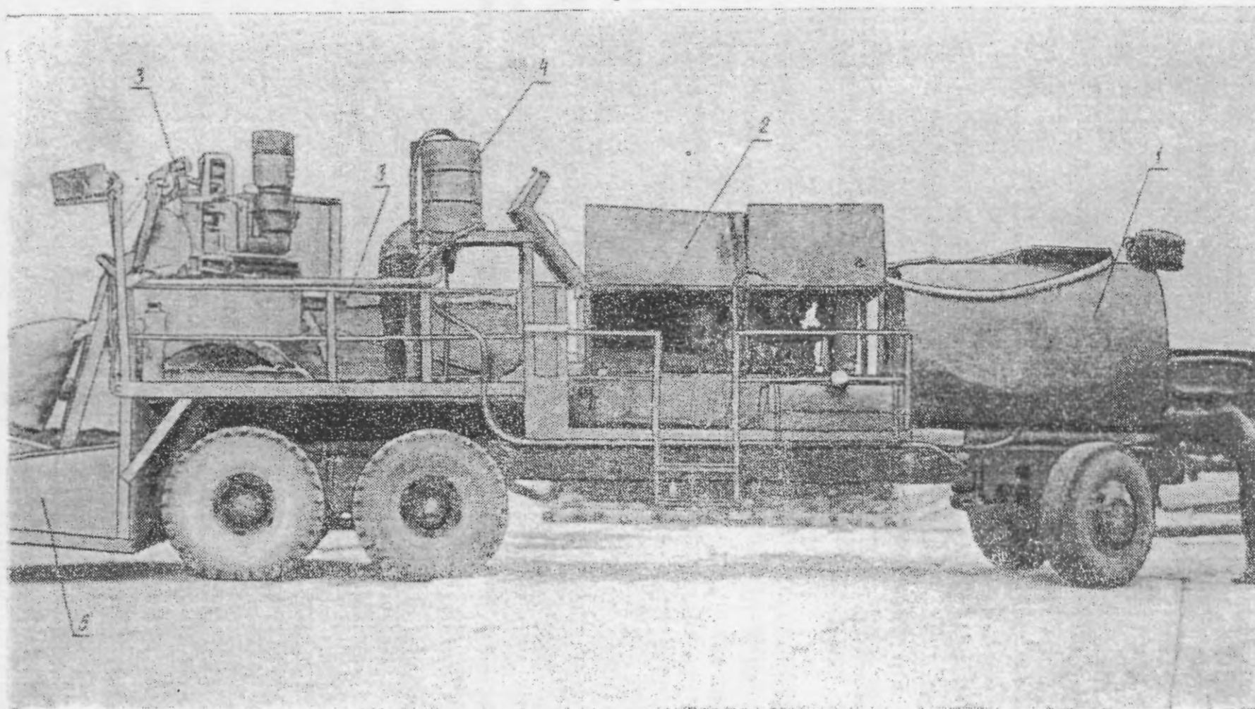
Рис. 3. Заливщик швов:
