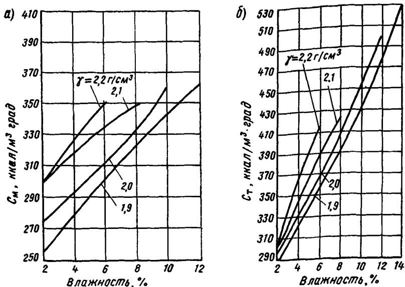
Рис. 21 Графики для определения объемной теплоемкости гравийно-песчаных смесей:
