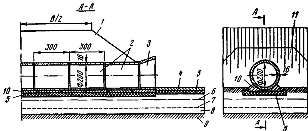
Рис. 6 Конструкция круглой трубы на водотоках с наледями:
