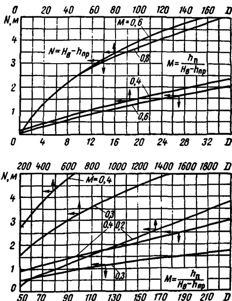
Рис. 1. Графики для определения параметра D при h_n : (H_b - h_{\text{пр}}) > 0,1
