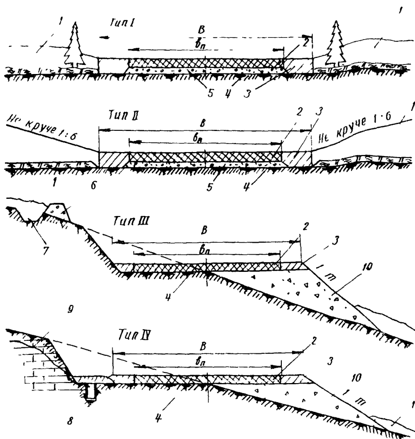
Рис.1. Поперечные профили автозимников на прочных грунтовых основаниях:
