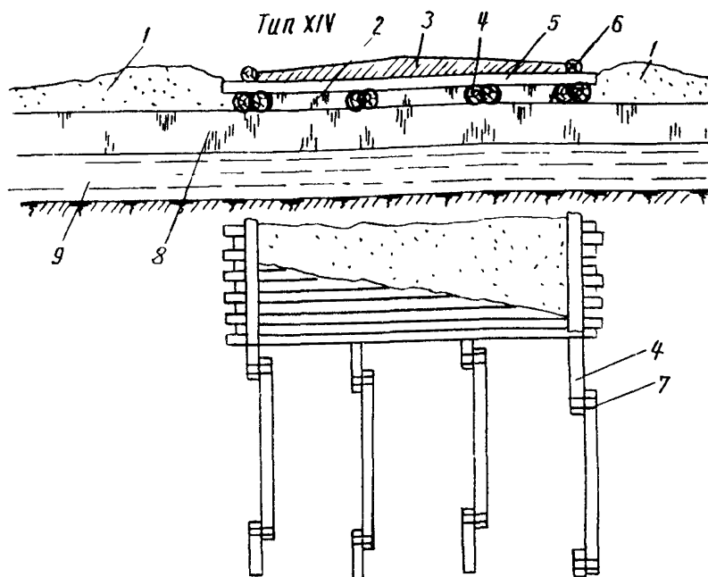
Рис.8. Конструкция "плавающей" дерево-ледяной переправы: 1-валик из снега; 2-намороженный слой льда; 3-грунтовая за- сыпка; 4-продольные лежни: d = 20-22\text{см} ; 5-сплошной сланевый настил из тонкомерной древесины d = 12-16\text{см} ; 6-колесоотбой- ные брусья d = 22-24\text{см} ; 7-проволочная скрутка d = 8\text{мм} ; 8-ес- тественный ледяной покров; 9-вода
