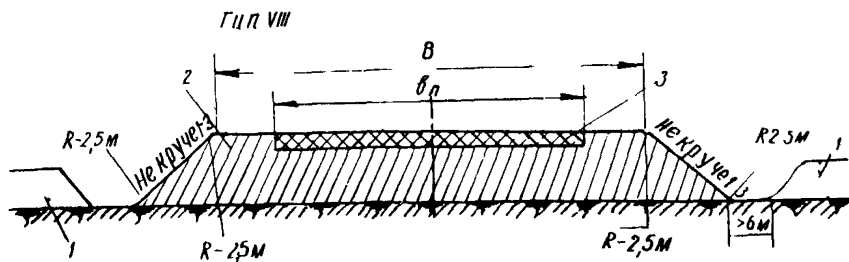
Рис.4. Поперечный профиль автозимника в насыпи из снега 1-снеговой покров; 2-насыпь из уплотненного снега; 3-оледенен- ный слой снега на проезжей части или настил из тонкомерной древесины, веток, сучьев и т.п.
