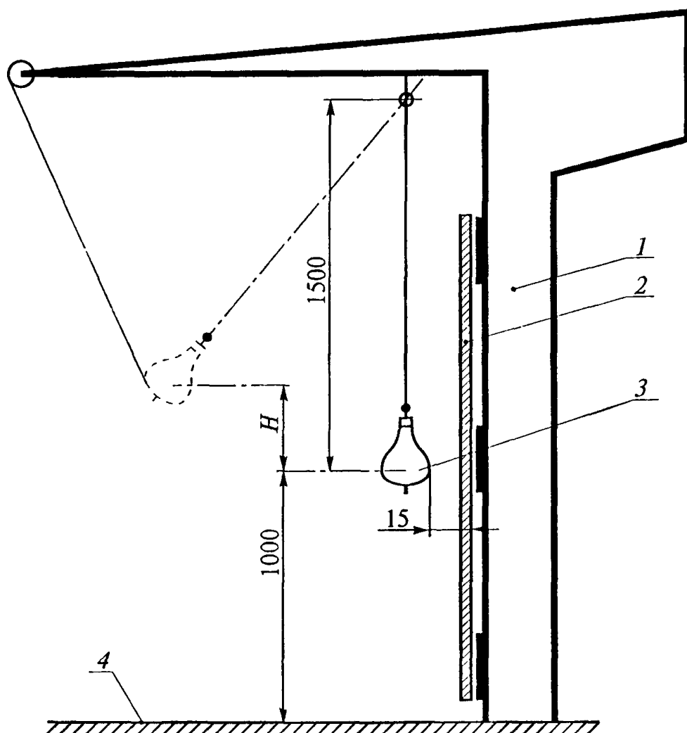
Рис. 1. Испытательный стенд:
