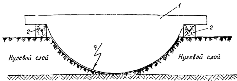
Рис. 3. Схема установки шаблона для вырезки ложа в нулевом слое:
