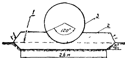
Рис. 2. Устройство песчано-гравийного основания под трубу:
