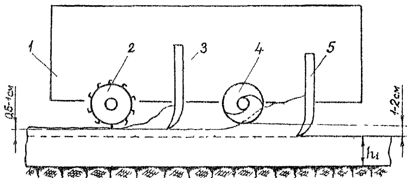
Рис.4. Установка рабочих органов профилировщика для чистовой планировки основания
