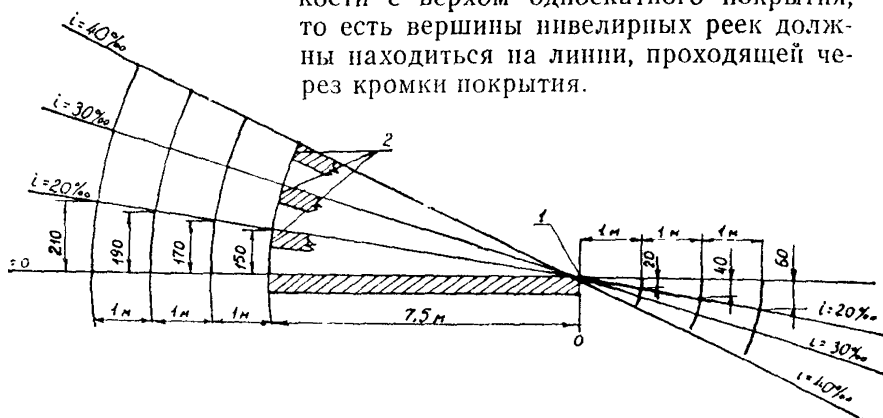
Рис. 4. Схема вертикальной разбивки виража для вычисления отметок нивелирных реек:
