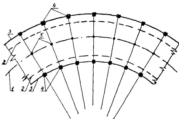
Рис. 5. Расположение нивелирных реек в плане на кривой виража:
