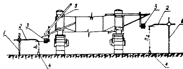
Рис. 7. Установка копирных струн в разных уровнях:
