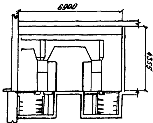
Разрез 1-1
