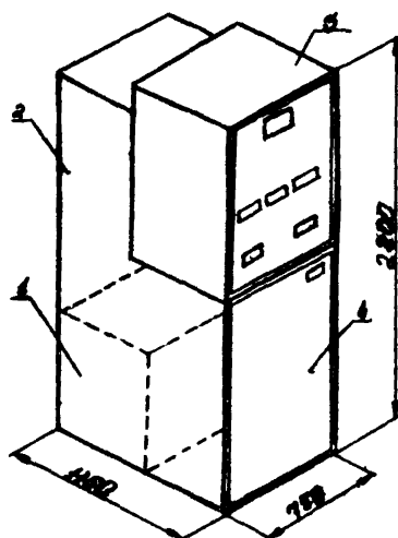
Рис. 2. Шкаф КРУ серии К-ІО4:
