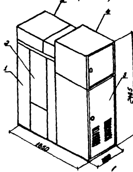
Рис.3. Шкафы КРУ серии КЗ-6, КЗ-6С (КЗЭ-6, КЗЭ-6С) и серии КЗ-ІО:
