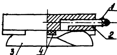
Рис. 7. Опора на воздушной подушке ОВП-1,6:
