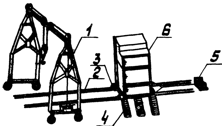
Рис. 6. Комплекс механизмов КМБ:
