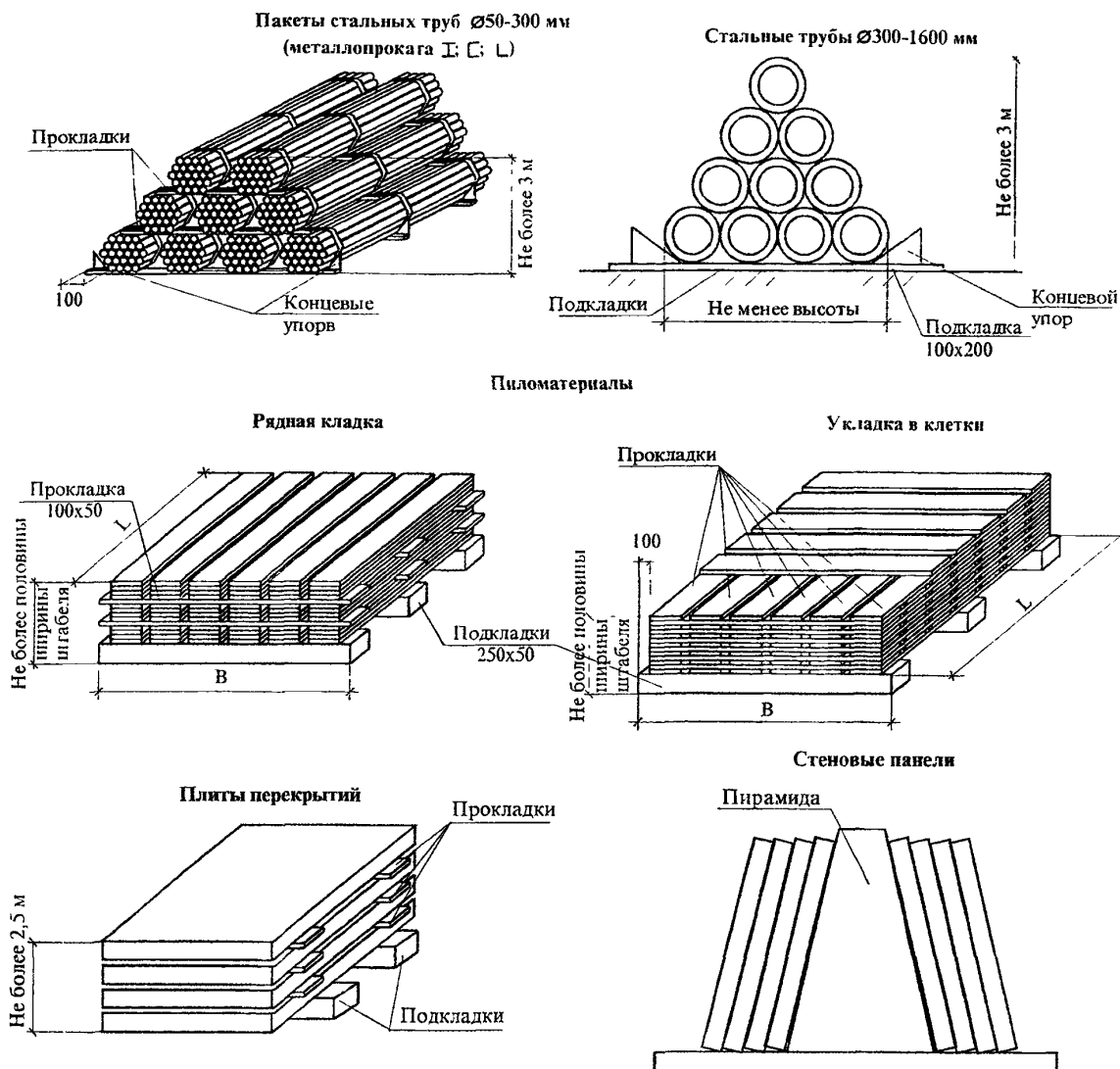
Рисунок 7 – Примеры складирования материалов, изделий и конструкций
