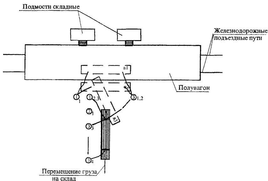
Рисунок 2 – Технологическая схема разгрузки полувагонов
