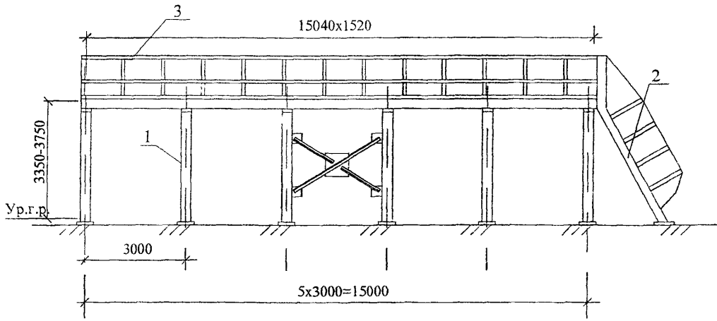
1 — стойки, 2 — лестница; 3 — ограждение
