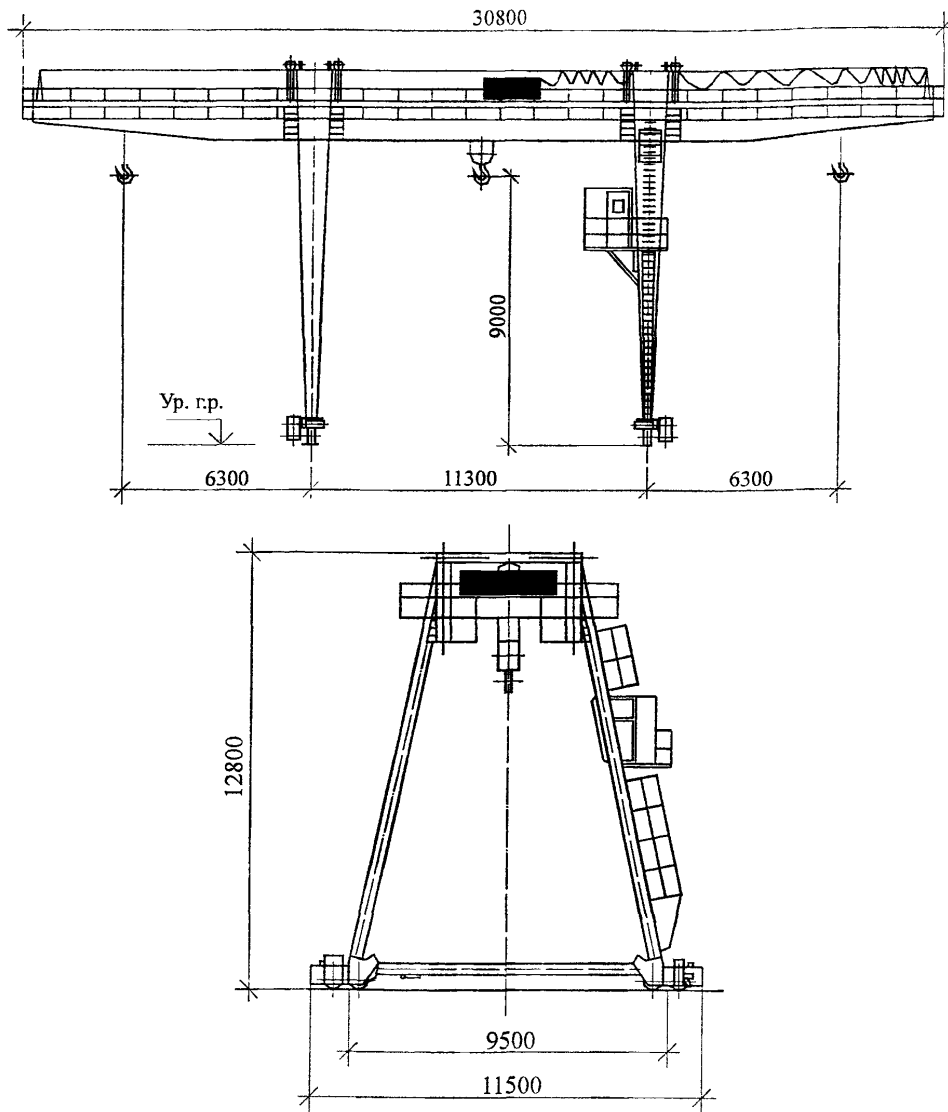
Рисунок 1 – Общий вид козлового крана КК 20-11,3-9
