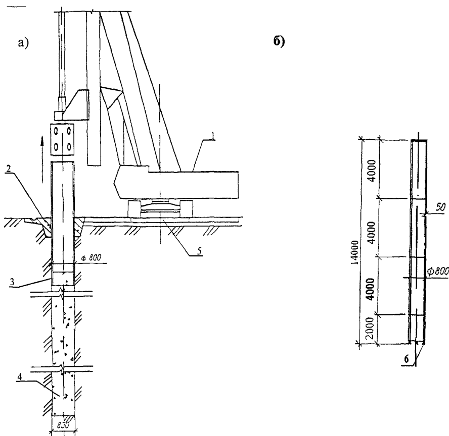
а – схема извлечения обсадной трубы; б – применяемые инвентарные секции обсадной трубы для скважины глубиной 14 м; 1 – буровая машина; 2 – форшакта; 3 – обсадная труба; 4 – бетонная смесь; 5 – плита дорожная; 6 – режущий наконечник инвентарной обсадной трубы.
