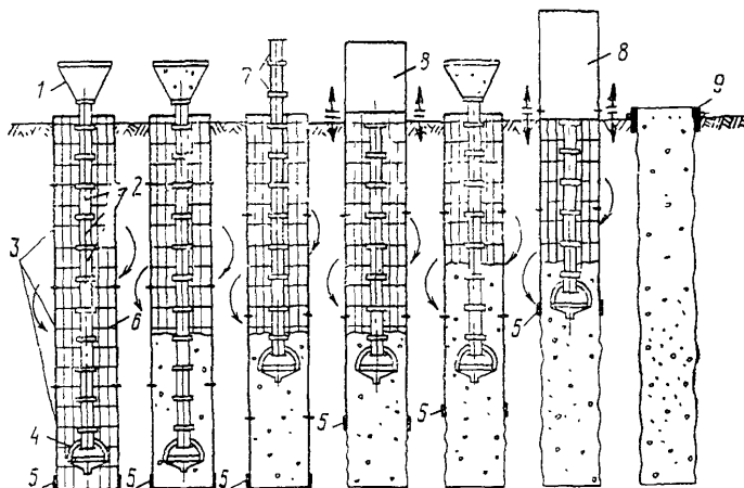
Рисунок 7 – Технологическая схема бетонирования сваи
