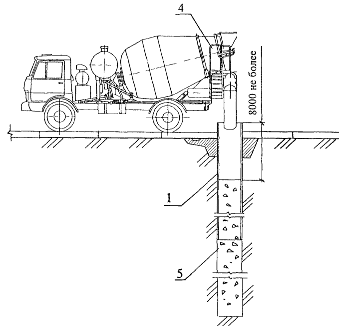
Рисунок 5 – Укладка бетонной смеси в скважину
