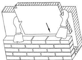
1 Установка пенополистирольных плит
