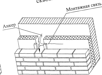
2 Протяжка монтажной связи сквозь анкер
