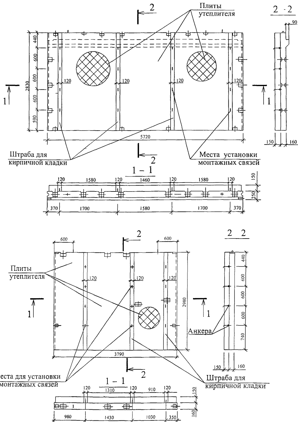
Рисунок 4 - Примеры раскладки теплоизоляционных пенополистирольных плит
