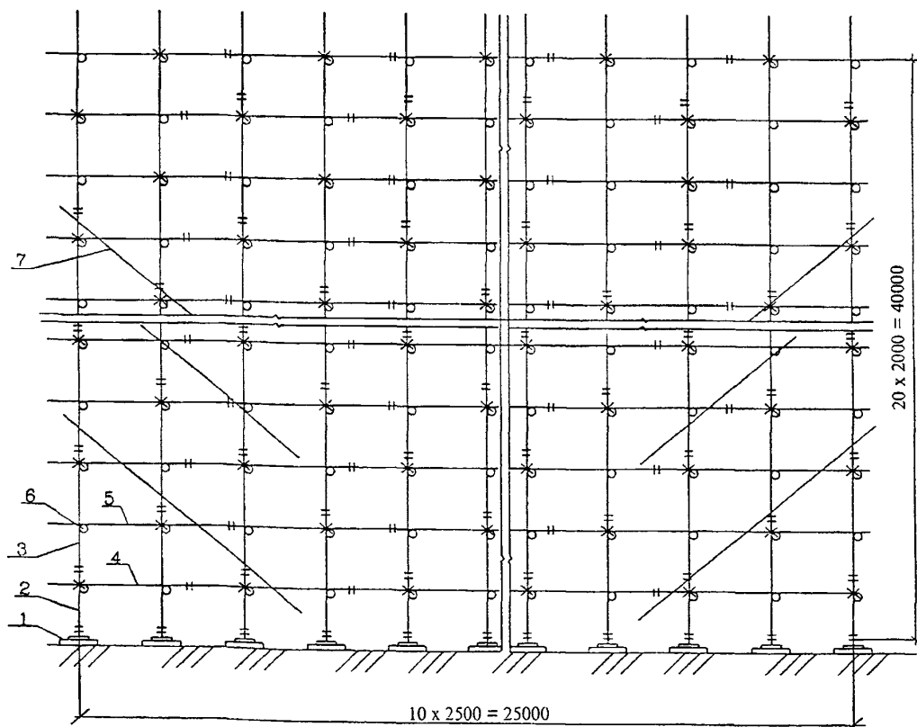
Рисунок 1 — Схема установки лесов по наружному ряду стоек
