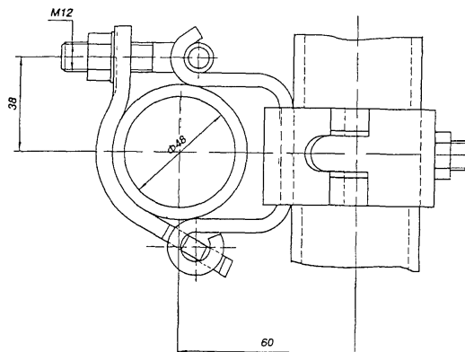
Рисунок 20 – Хомут неповоротный
