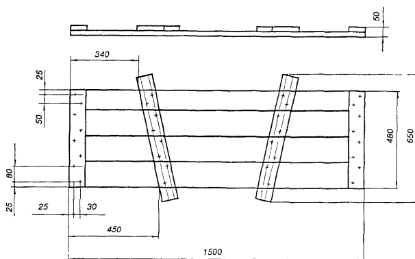
Рисунок 22 – Щит настила
