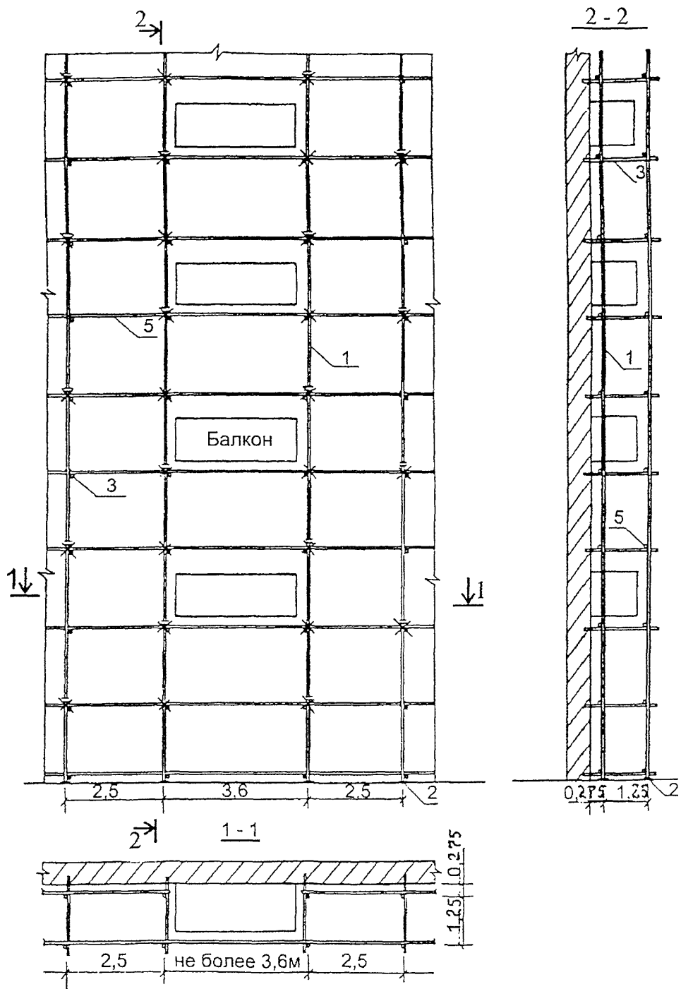
Рисунок 6 — Схема крепления лесов при наличии балконов
