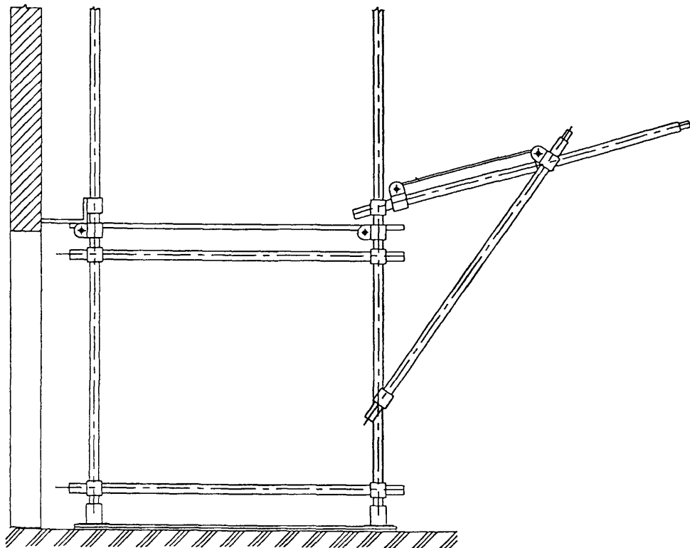
Рисунок 12 – Козырек
