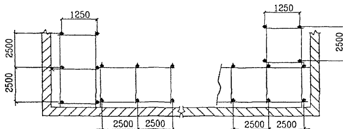
Рисунок 5 — Схемы установки лесов при различной конфигурации зданий
