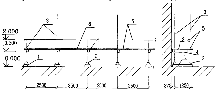
7) Схема раскладки щитов настила первого монтажного яруса на отм. 0,500
