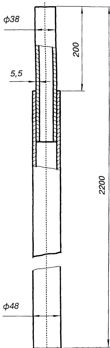
Рисунок 17 – Стойки лесов
