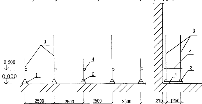
5) Схема установки продольных связей на отм. 0,500 (1 ярус)
