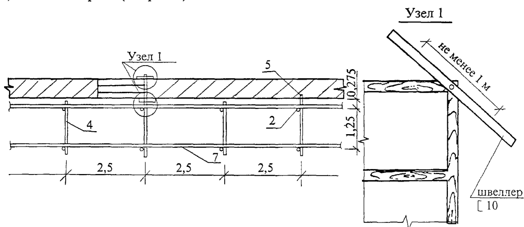
Рисунок 10 — Схема крепления лесов при наличии оконных проемов
