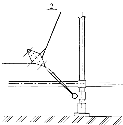
Рисунок 3 — Схема подъема груза лебедкой
