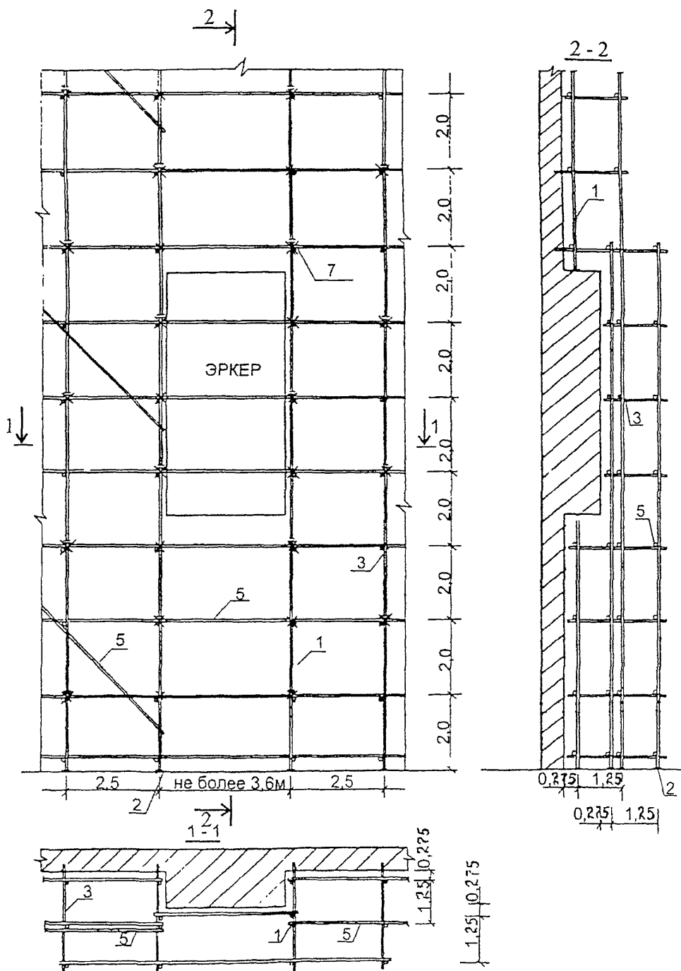
Рисунок 9 — Схемы установки лесов при наличии эркера
