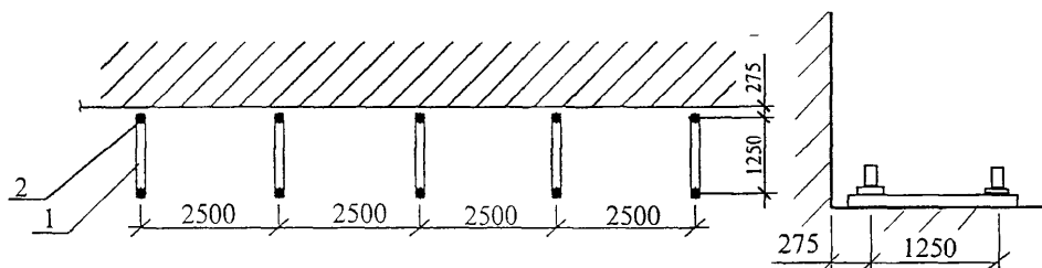
2) Схема установки башмаков (1 ярус)
