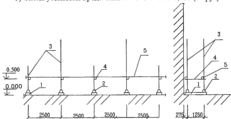
5) Схема установки продольных связей на отм. 0,500 (1 ярус)
