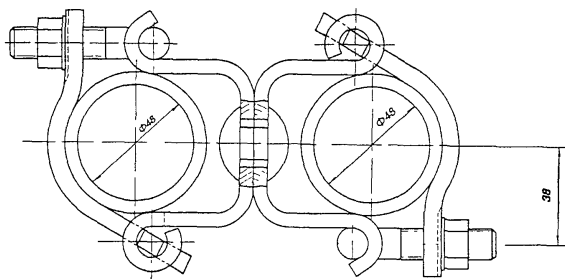
Рисунок 21 – Хомут поворотный
