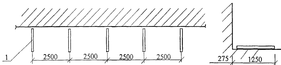
2) Схема установки башмаков (1 ярус)
