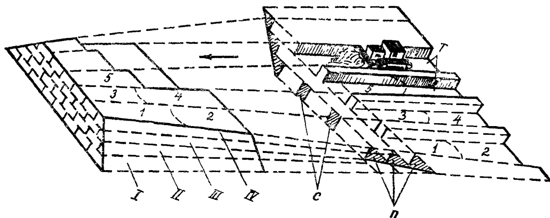
Рис 6 Ярусно-траншейная схема разработки бульдозером грунта в выемке с перемещением его в насыпь:
