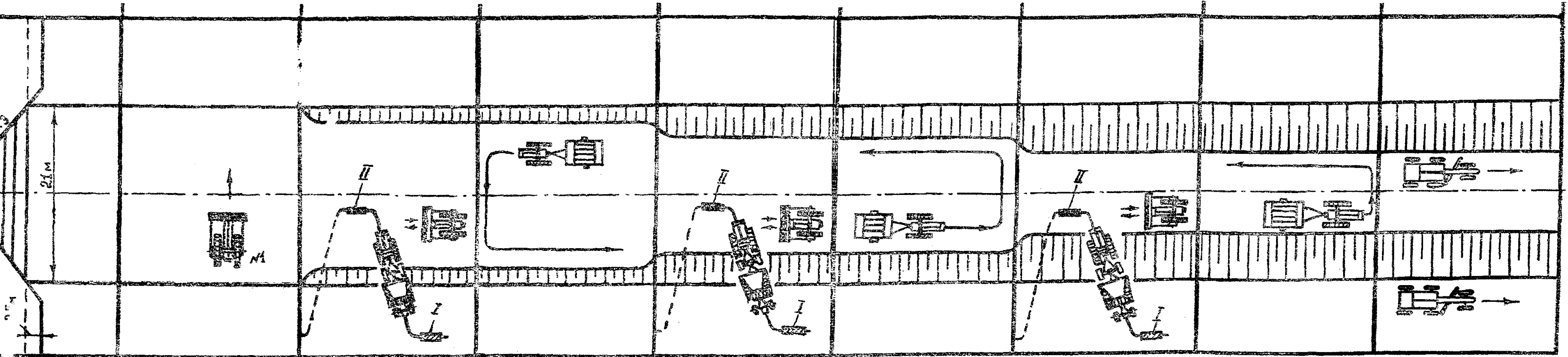
Рис. 7. Технологическая схема возведения земляного полотна скрепером по зигзагообразной схеме: I — набор грунта; II — разгрузка грунта.
