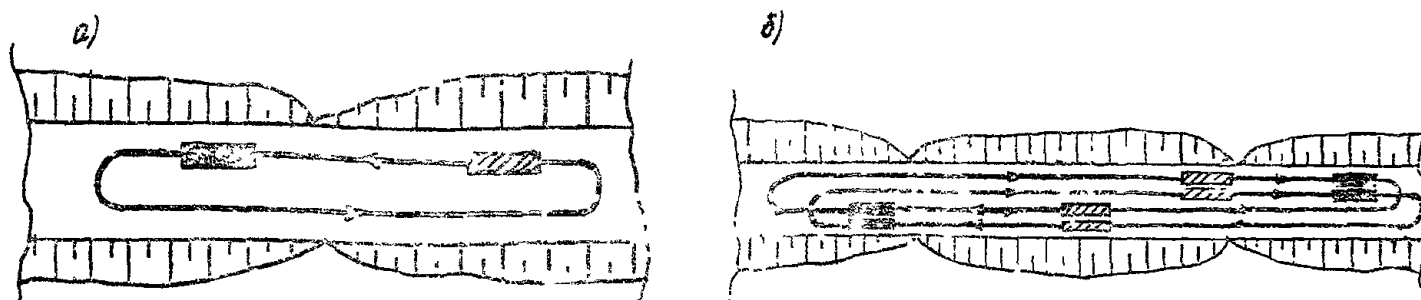
Рис. 9. Схема движения скрепера при разработке грунта в выемке с перемещением его в насыпь: а) из выемки в насыпь; б) из выемки в две насыпи
