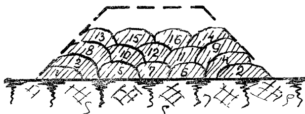
Рис 6 Последовательность отсыпки грунта скрепером
