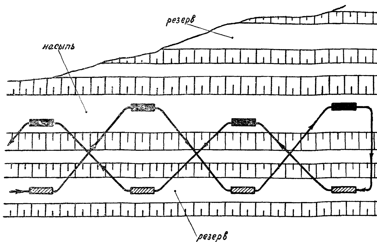
Рис 5 Зигзагообразная схема перемещения грунта:
