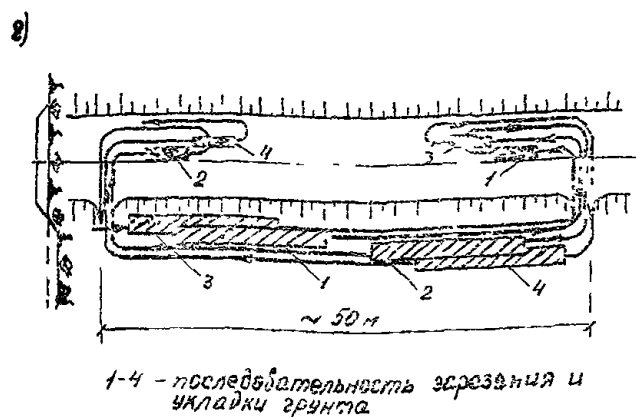
Рис. 8. Схемы движения скреперов при разработке грунта:
