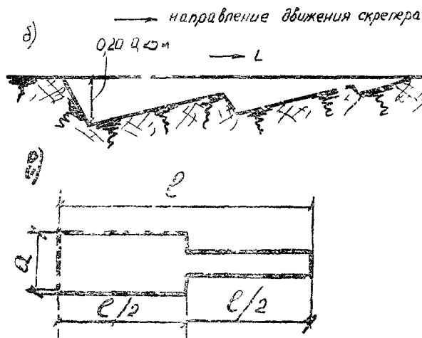
Рис 1 Шахматная схема набора грунта:
