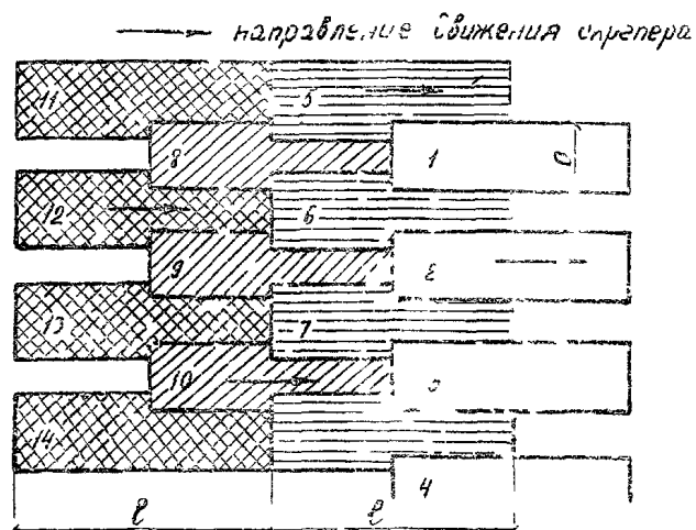
Рис 1 Шахматная схема набора грунта:
