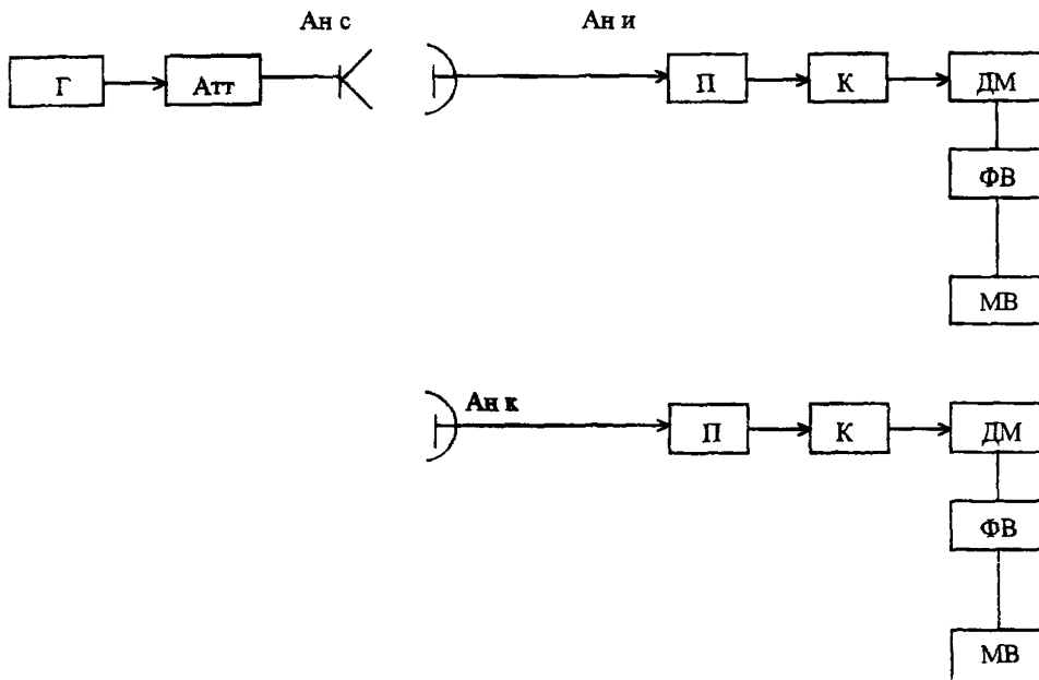
Рисунок 6 - Схема измерения добротности станции
