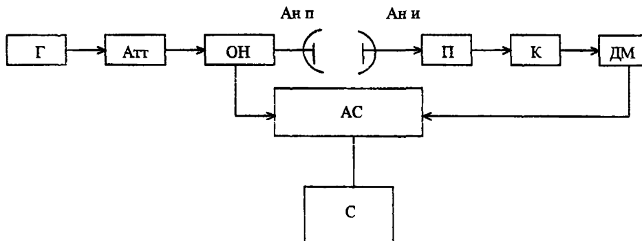
Рисунок 4 - Схема для измерений уровня боковых лепестков антенны
