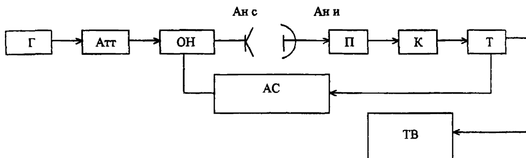
Рисунок 2 - Схема для определения диапазона принимаемых частот
