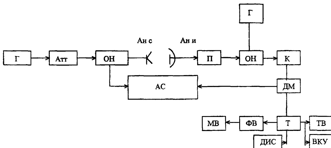
Рисунок 8 - Схема для измерений порогового отношения сигнал/шум
