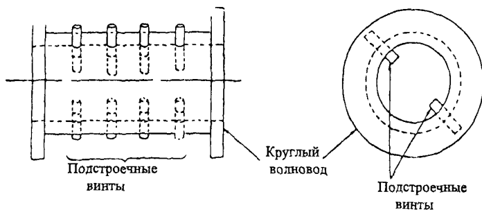
Рисунок А 3 - Структура кругового поляризатора
