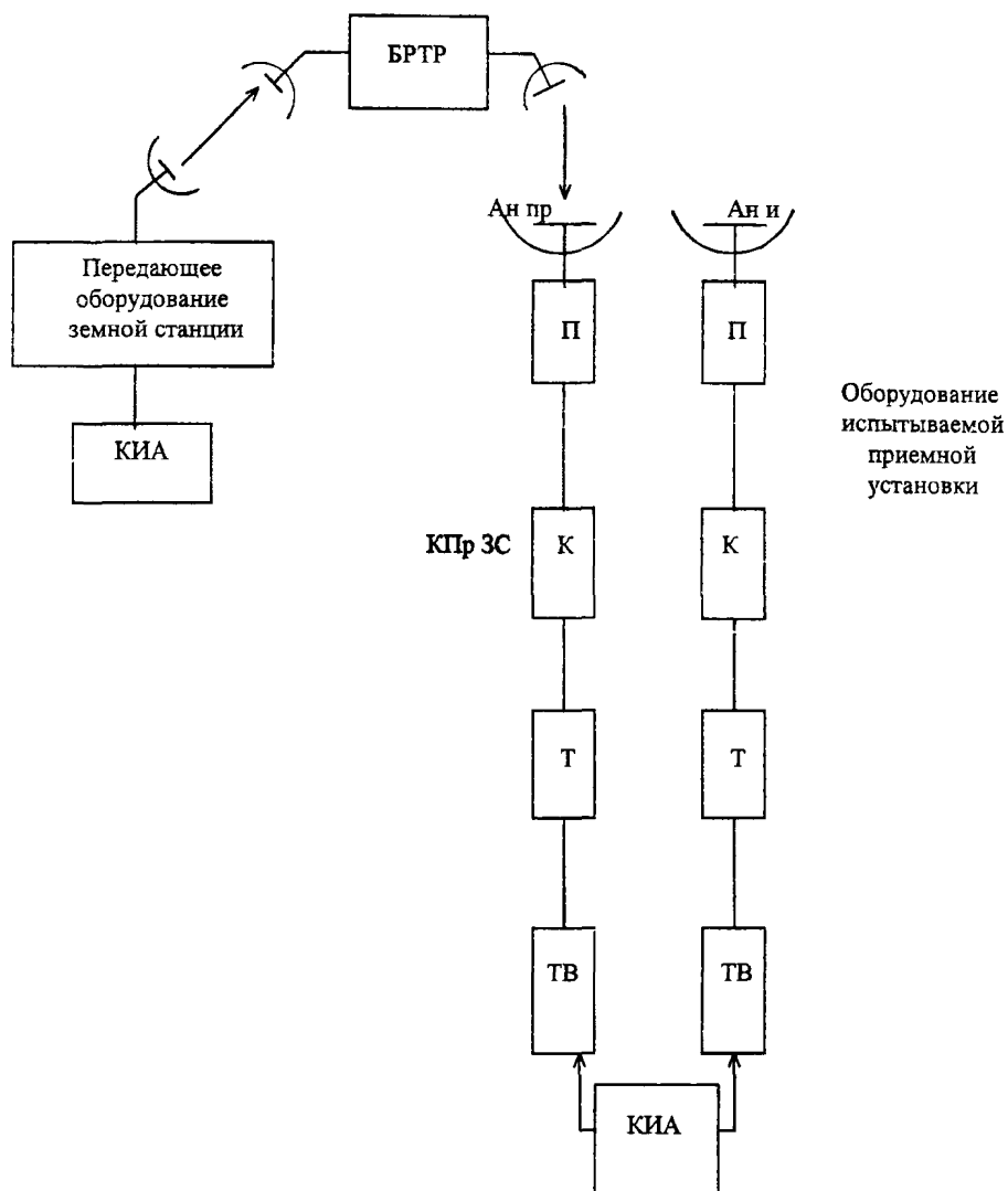
Рисунок 1 - Схема измерения параметров оборудования испытываемой приемной установки методом сравнения в составе космического сегмента
