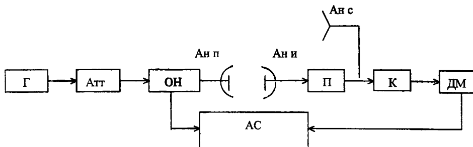
Рисунок 3 - Схема для измерения усиления антенны
