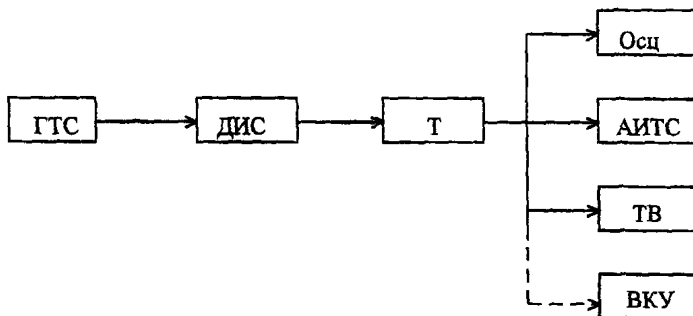
Рисунок 9 - Схема измерения АЧХ тракта изображения, дифференциального
