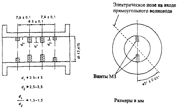
Рисунок А 3 - Структура кругового поляризатора
