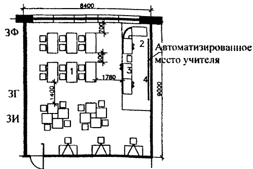
Рис. 6 Учебный кабинет универсальный (КТ-I). Обозначение зон кабинетов: ЗФ-зона фронтальных работ; ЗГ - зона групповой работы; ЗИ-зона индивидуальной работы; ЗЛ- зона лаборантской
