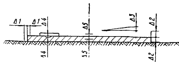
Схема цементогрунтового основания с указанием предельных отклонений
