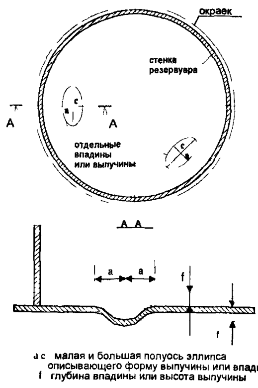
Фиг. 5-5. Отдельные впадины или выпучины на дне
