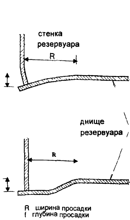
Фиг 5-3 Просадка края
