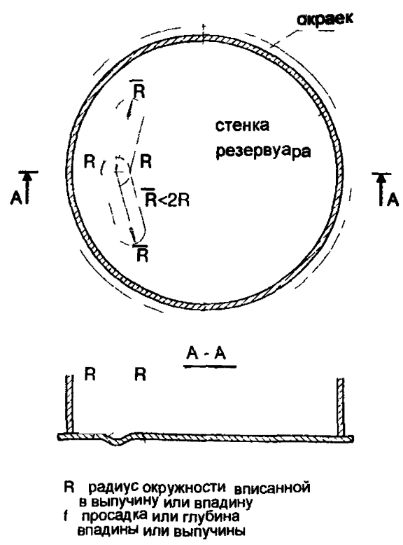
Фиг 5-4 Просадка дна вблизи стенки
