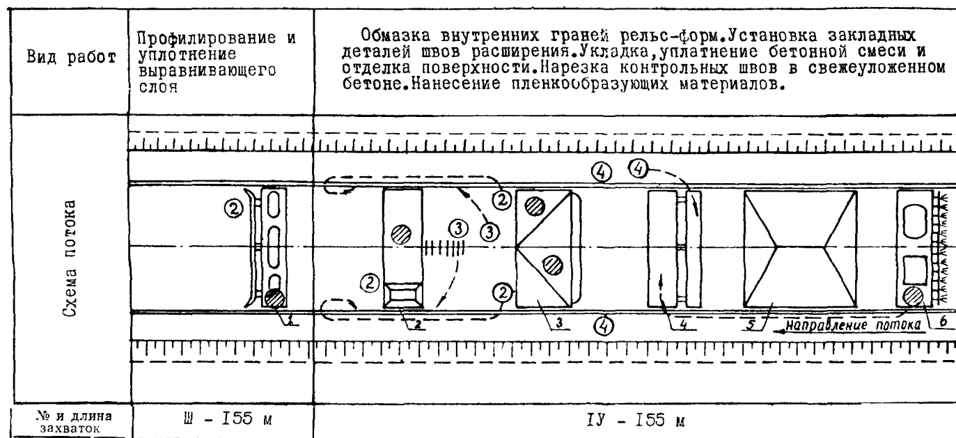
Рис. 6. Технологическая схема устройства цементобетонного покрытия:
