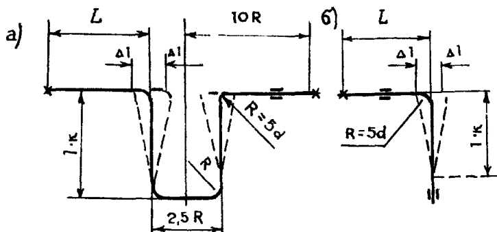
Рис. 1. Устройство компенсаторов П-образного (а), Г-образного (б)
