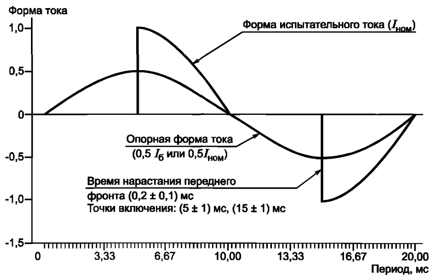
Рисунок А.5 — Форма тока при фазовом управлении
