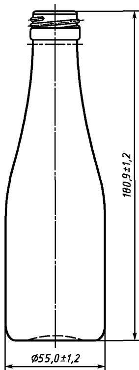
Венчик горловины — тип В-28Д. Номинальная вместимость, см 3 , — 200. Полная вместимость, см 3 , — 215 ± 6.
