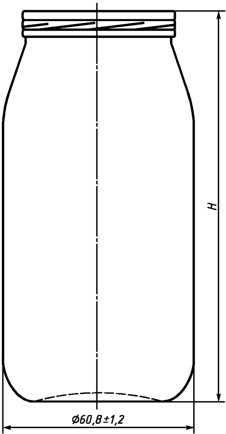
Венчики горловины: тип II-51 при H = (118,5 \pm 1,5) мм; тип III-53 при H = (124,8 \pm 1,5) мм. Номинальная вместимость, см 3 , — 230. Полная вместимость, см 3 , — 250 \pm 10 .
