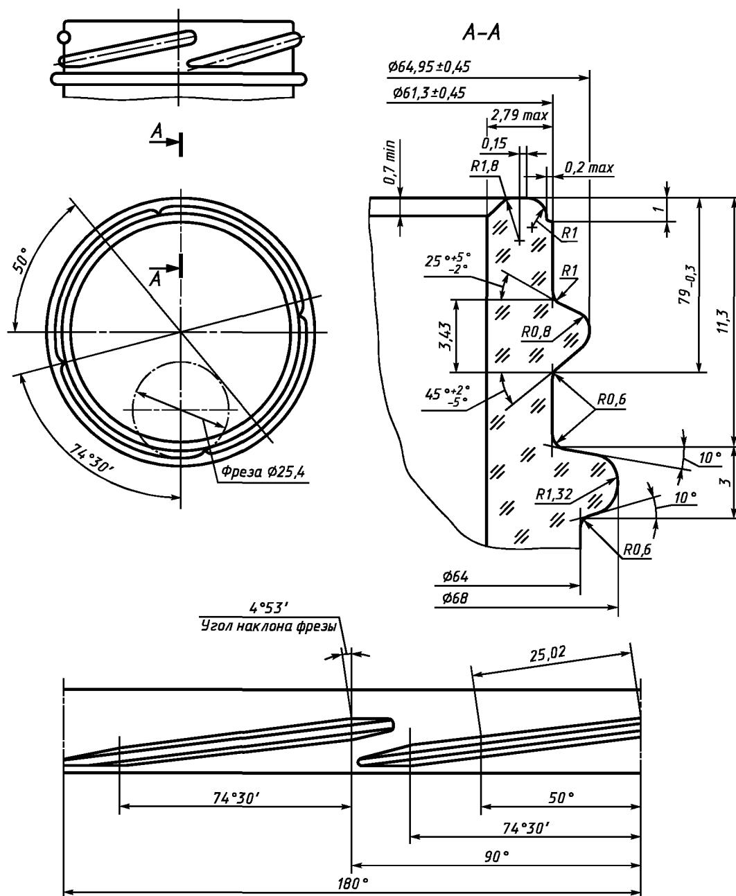
Рисунок 11 — Венчик типа III-66
