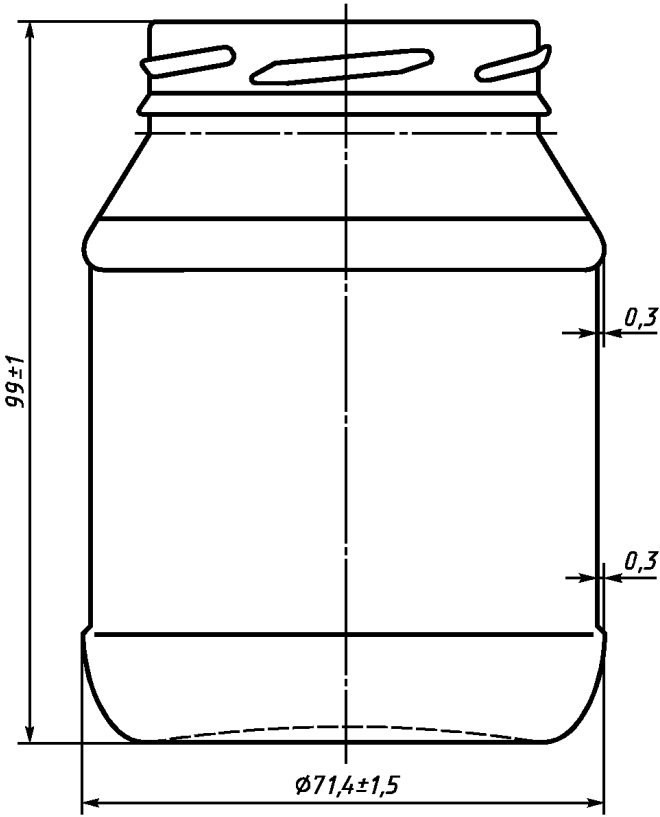
Венчик горловины — тип III-58. Номинальная вместимость, см 3 , — 250. Полная вместимость, см 3 , — 270 \pm 8 .
