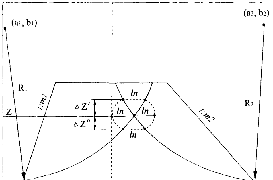
Рис.7. Зона взаимного влияния на устойчивость армированной насыпи потенциальных поверхностей обрушения ее левого и правого откосов.
