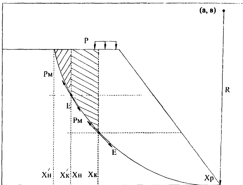
Рис.4. Схема определения оптимального места расположения в теле откоса горизонтов армирования.
