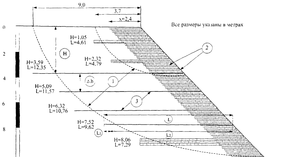
Рис. 11. Схема армирования насыпи с углом скольжения откоса 45^\circ 1 - расчетные поверхности скольжения; 2 - георешетки "Прудон - 494" 3 - геотекстильный материал"
