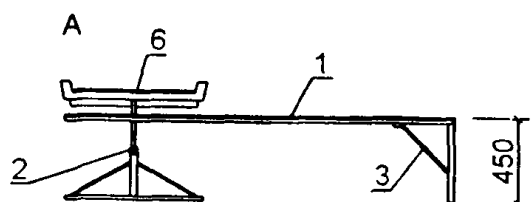
Скамья для занятий тяжелой атлетикой
