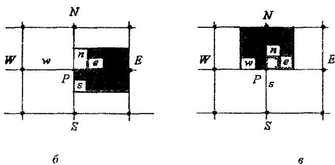
Рис II 2 Шаблоны контрольных объемов а - для основных узлов конечно-разностной сетки, б - для проекции скорости на ось OX , в - для проекции скорости на ось OY
