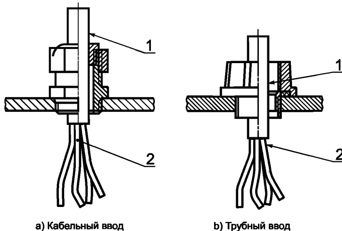
1 — место ввода кабеля; 2 — место разделки жил кабеля
