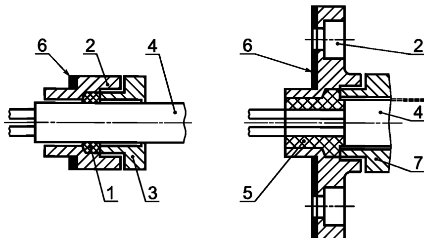
1 — уплотнительное кольцо; 2 — корпус ввода; 3 — нажимная деталь; 4 — кабель; 5 — герметизирующий компаунд; 6 — уплотнение; 7 — деталь, фиксирующая компаунд
