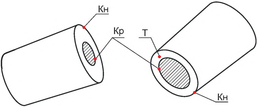
Рисунок В.6 — Стаканчик для изложниц
