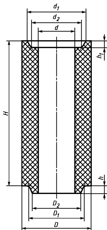
Рисунок 2 — Центровая трубка
