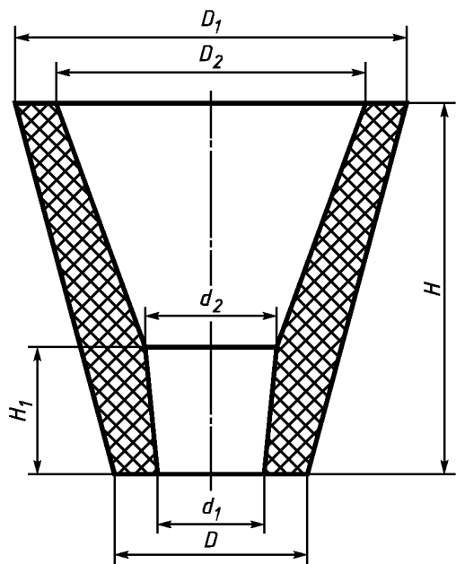
Рисунок 23 — Промежуточная воронка
