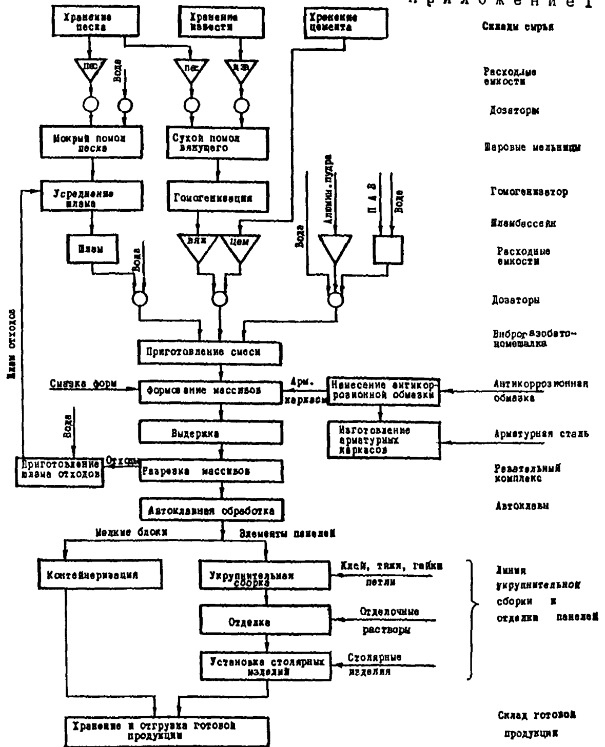
ПРИНЦИПИАЛЬНАЯ ТЕХНОЛОГИЧЕСКАЯ СХЕМА ИЗГОТОВЛЕНИЯ ИЗДЕЛИЙ ИЗ ЯЧЕЙСТОГО БЕТОНА ПО РЕЗАТЕЛЬНОЙ ТЕХНОЛОГИИ
