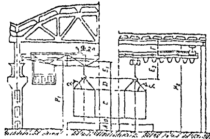
Рис. 12. Расчет высоты по наиболее высокому изделию, ремонтному в цехе
