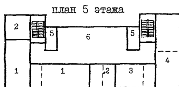
Рис. 4 Типологические схемы перепланировки и использования помещений существующего здания школы типа МЮ для проектируемой школы на 33 класса (825 учащихся)
