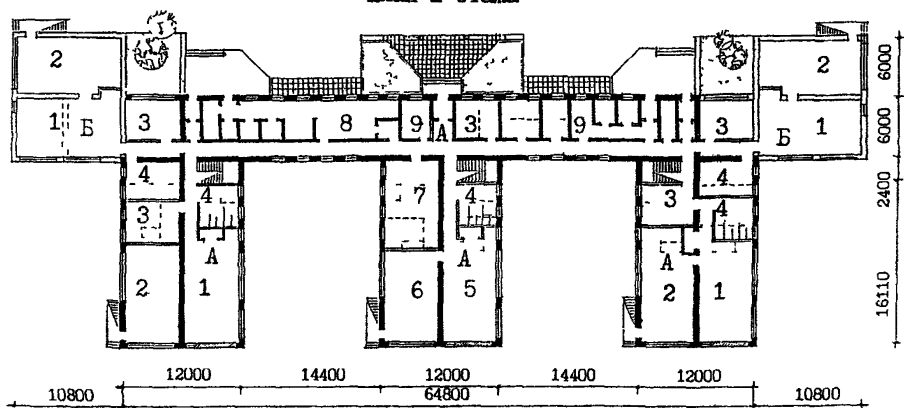
план 1 этажа
