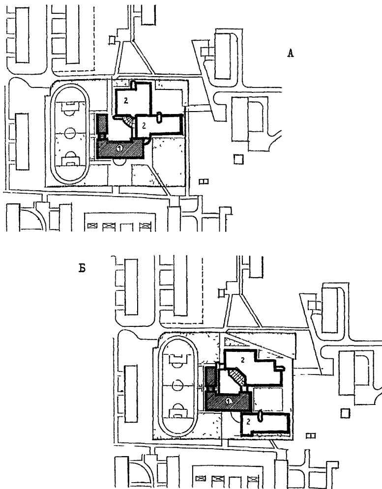
Рис. 11 Примеры генпланов участков с размещением пристраиваемых объемов к реконструируемым зданиям школ типа МЮ в квартале 81 Хорошево-Мневники.
