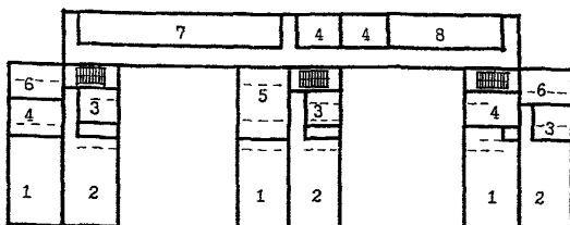
ПЛАН 1 этажа
