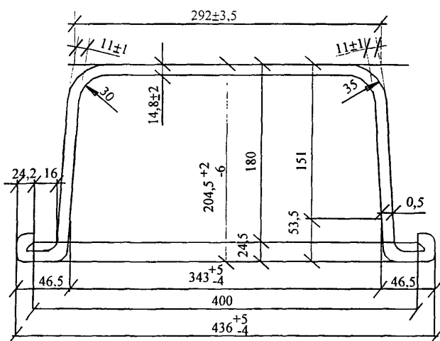
«Ларсен-ІУ»
