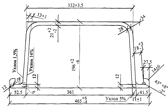
«Ларсен-У»
