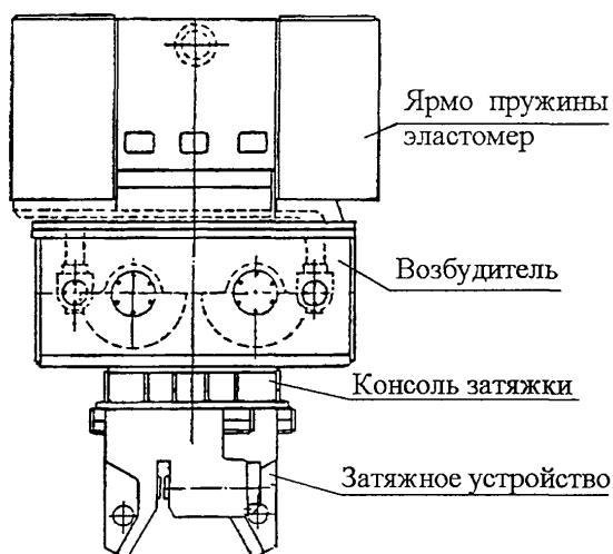
Рисунок 3 — Вибратор MS-25H
