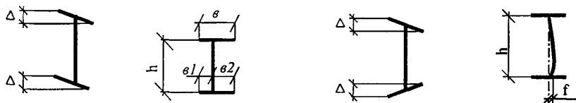
Рисунок 1 — Предельные отклонения по форме поперечного сечения.
