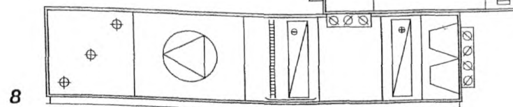
8. Приточно-вытяжная двухъярусная рециркуляционная установка с секцией пароувлажнения
