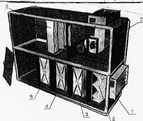
Рис. 2. Двухярусный*.
