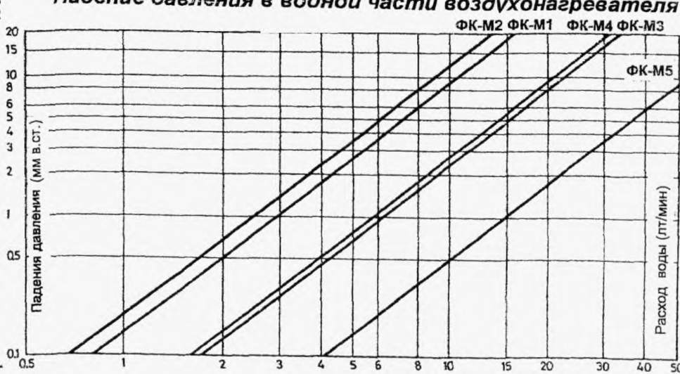
Падение давления в водной части воздушонагревателя
