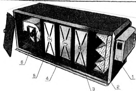
Рис. 1. Прямоточный*.
