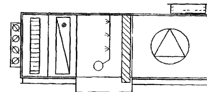
3 Кондиционер прямоточный с оросительной форсуноч- ной камерой
