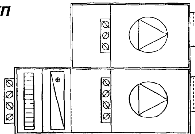
2 Приточная камера, с ре- зервным вентилятором (промежуточные камеры и резервный вентилятор мо- гут располагаться также в горизонтальной плоскости)
