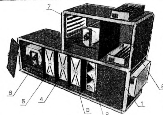
Рис. 3. Приточно-вытяжной*.
