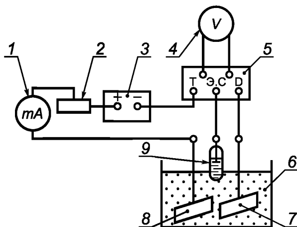
1 — миллиамперметр; 2 — регулируемое сопротивление; 3 — источник постоянного тока; 4 — вольтметр; 5 — прерыватель тока с клеммами для подключения электродов: Т — вспомогательного, Э — сравнения, D — рабочего; 6 — ячейка; 7 — рабочий электрод; 8 — вспомогательный электрод; 9 — электрод сравнения
