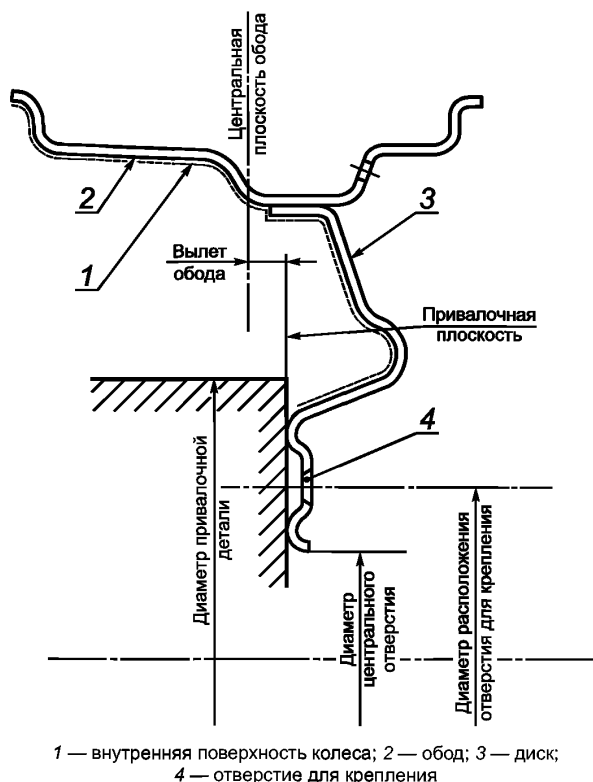
Рисунок 1 — Профиль колеса
