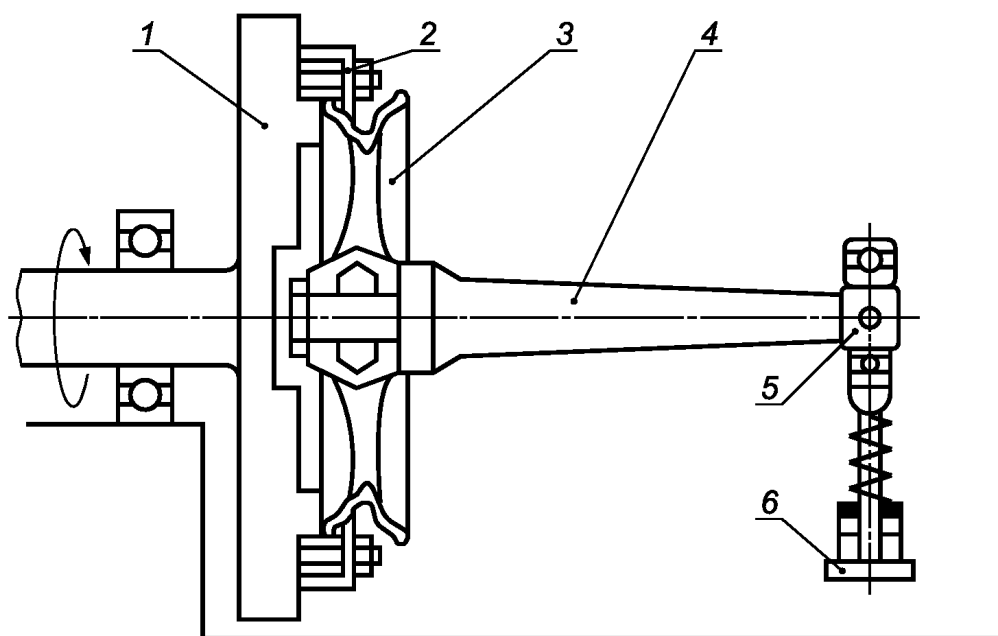
Рисунок Д.2 — Схема испытания под воздействием крутящего момента на подвижное колесо
