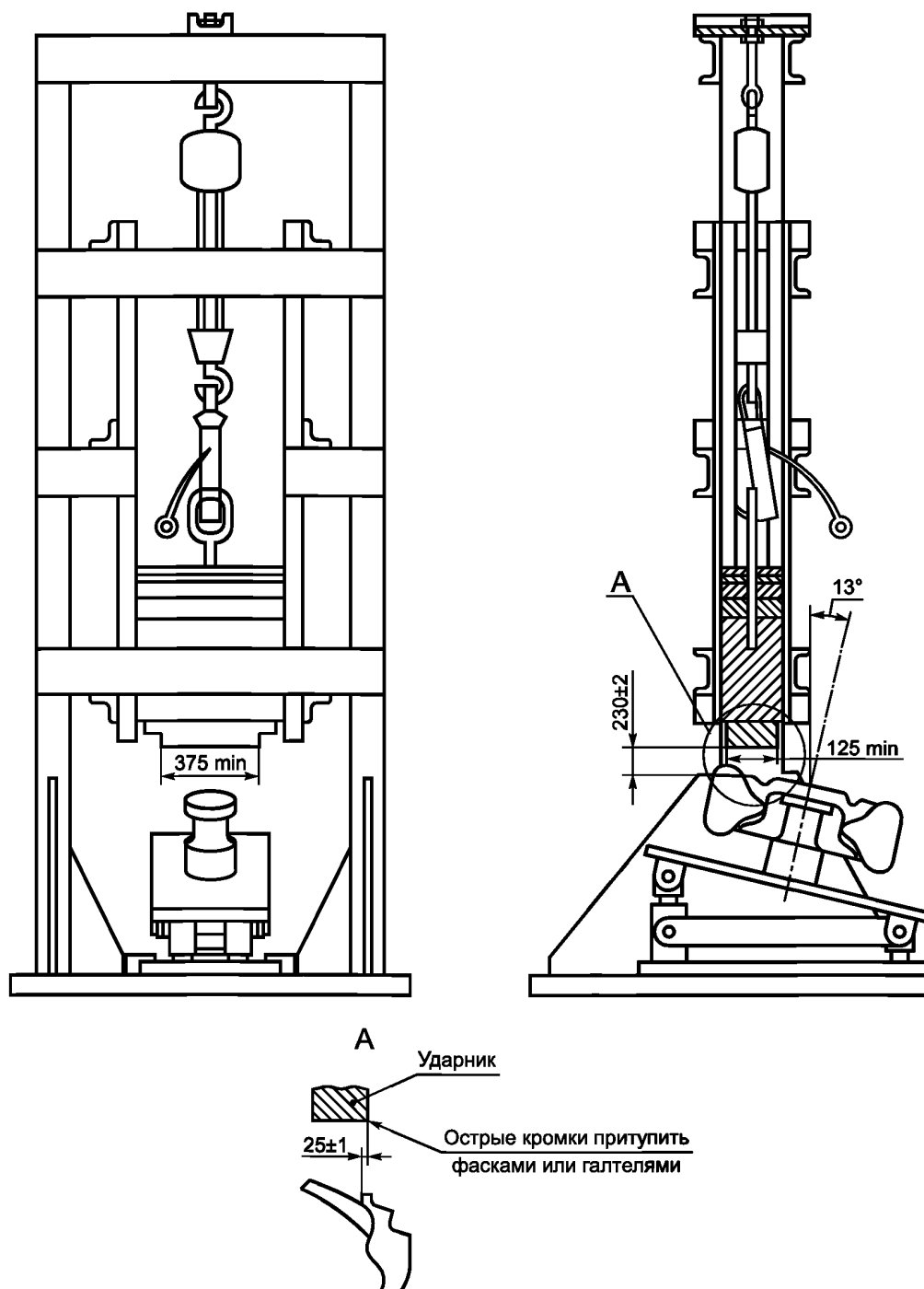
Рисунок И.1 — Стенд для определения сопротивления колеса удару под углом 13^\circ
