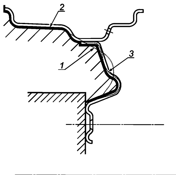
1 — профиль специального колеса внутри контура оригинального колеса; 2 — профиль поверхности внутреннего пространства колеса; 3 — профиль специального колеса снаружи контура оригинального колеса
