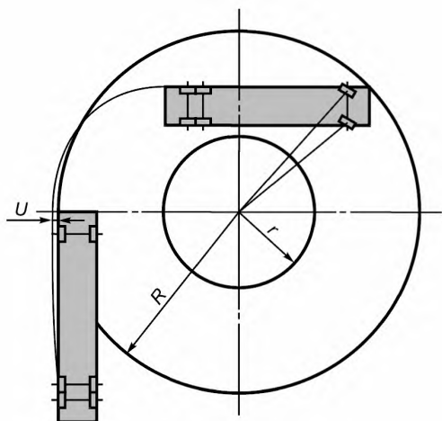
Рисунок 3 — Схема поворота трехосного транспортного средства
