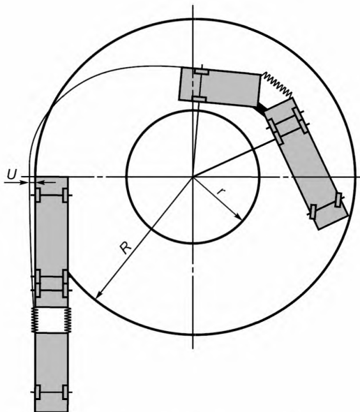
Рисунок 4 — Схема поворота сочлененного транспортного средства
