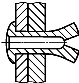
Рисунок 10 — Забивной штифт
