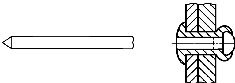
Рисунок 11 — Открытый конец
