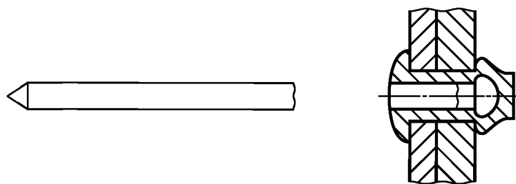
Рисунок 13 — Закрытый конец
