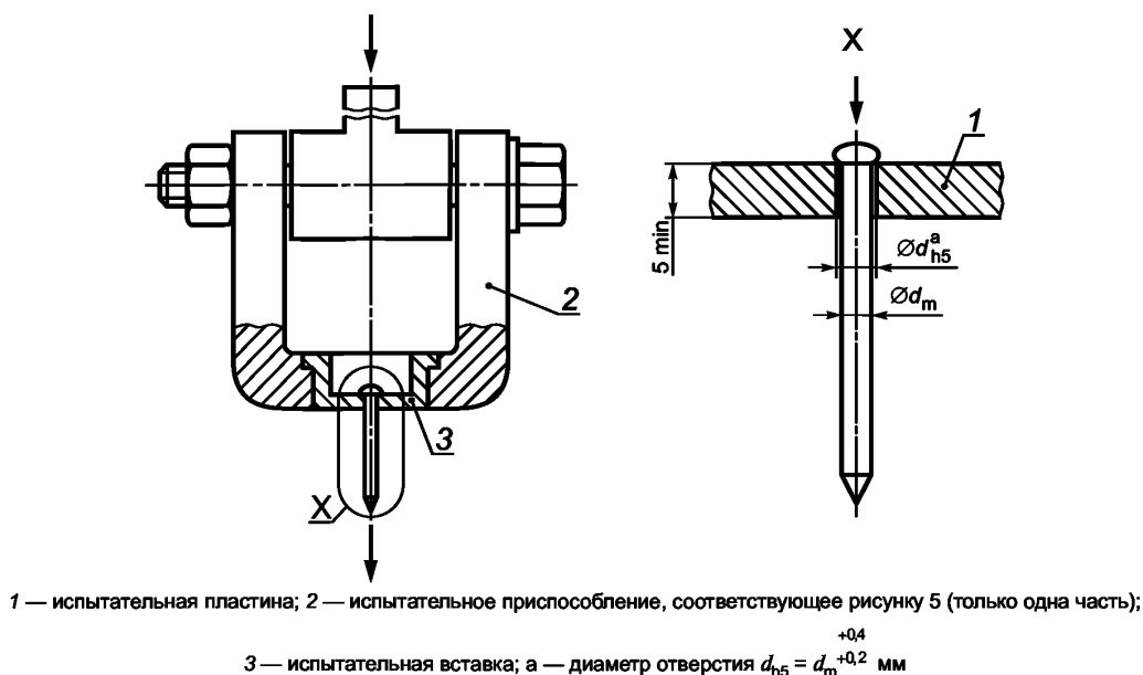
Рисунок 8 — Приспособление для испытания усилия разрыва сердечника
