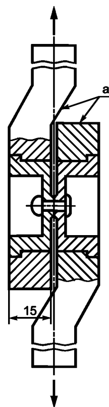
Рисунок 1 — Приспособление для обычных испытаний на срез
