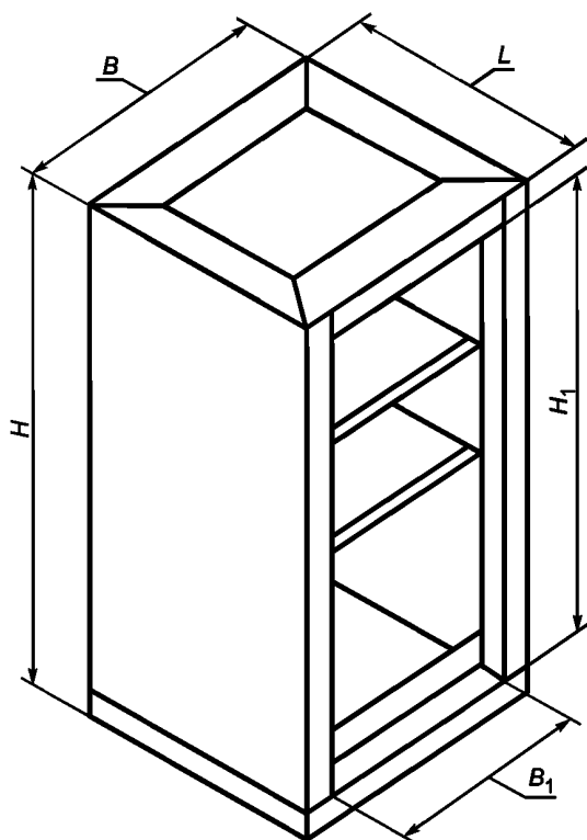
Рисунок 5 — Размеры корпусов СЭМ 3 на базе шкафа (стойки)
