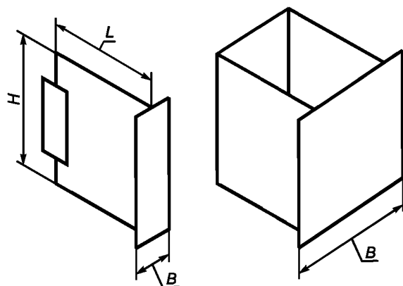
Рисунок 2 — Размеры корпусов СЭМ 1
