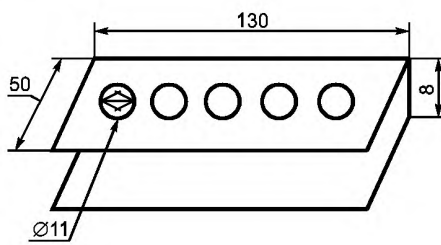
Рисунок 2 — Штатив для люминометрической кюветы
