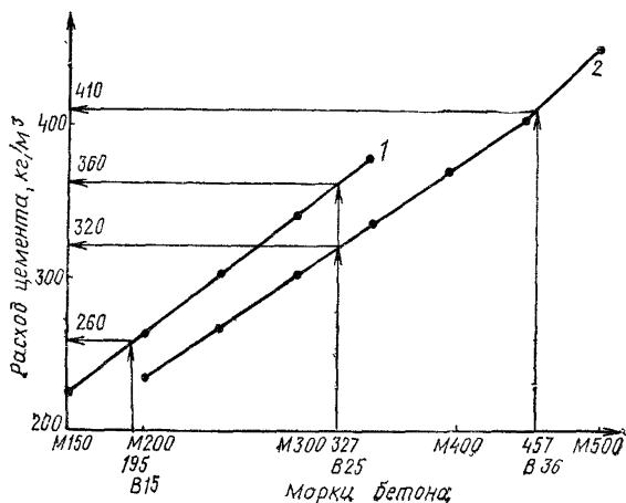
График зависимости расхода цемента марки 400 (1) и марки 500 (2) от марки бетона
