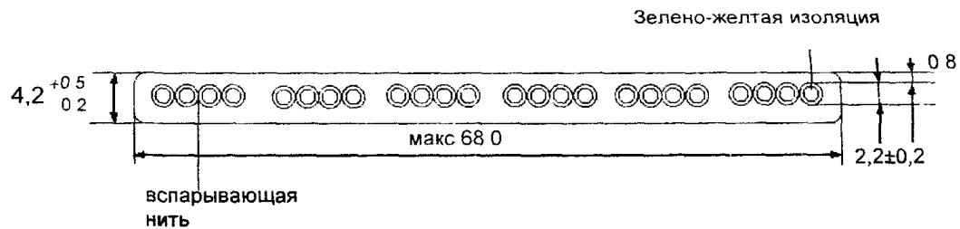
Рисунок 1 – Кабель КПЛ-24
