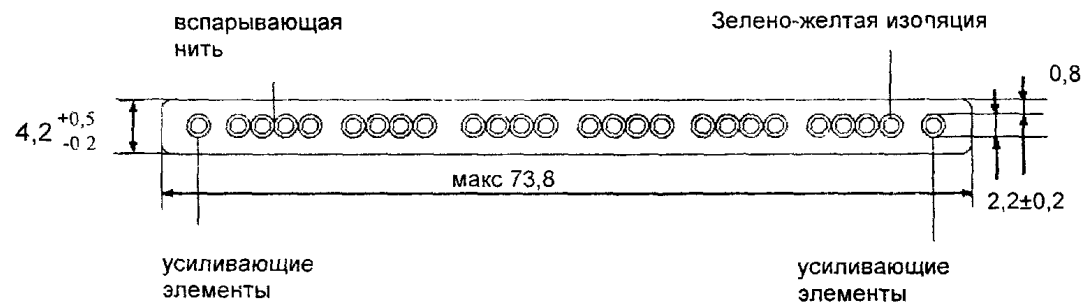
Рисунок 2 – Кабель КПЛУ-24
