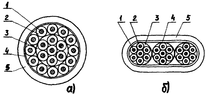
Рисунок 1 - Кабели управления круглой (а) и плоской (б) формы 1 - токопроводящая жила; 2 - изоляция; 3 - сердечник; 4 - скрепляющая обмотка; 5 - защитная оболочка.
