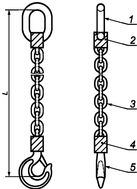
а) Смонтированная стропальная цепь из одного жгута
