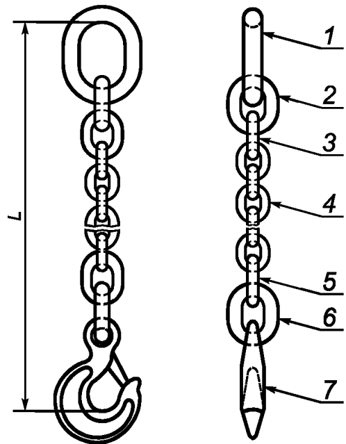
б) Сварная стропальная цепь из одного жгута
