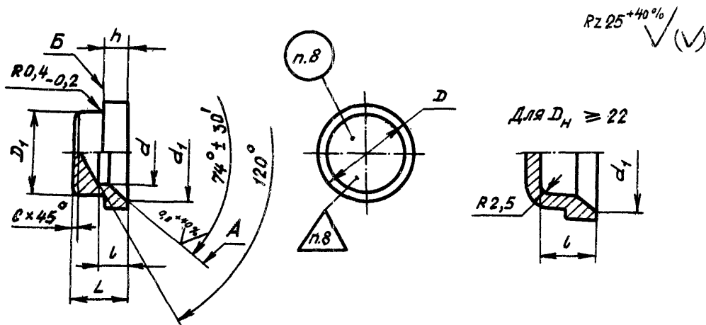
Размеры, мм
